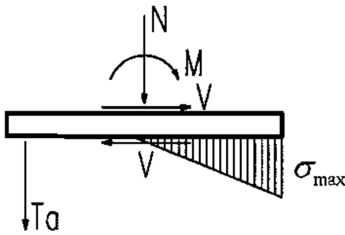
图4.2.2 计算简图
