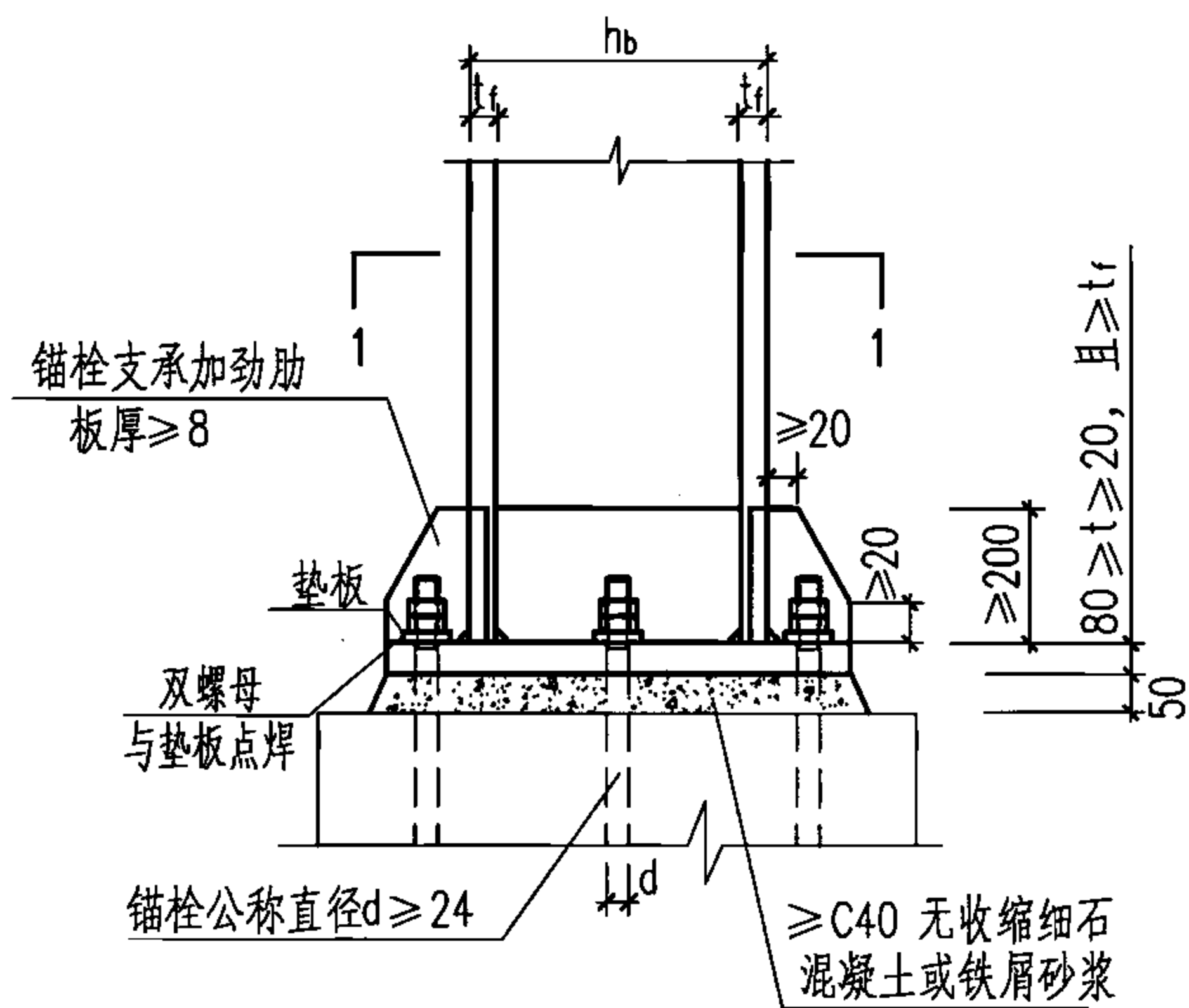
无靴梁板式柱脚(二)
