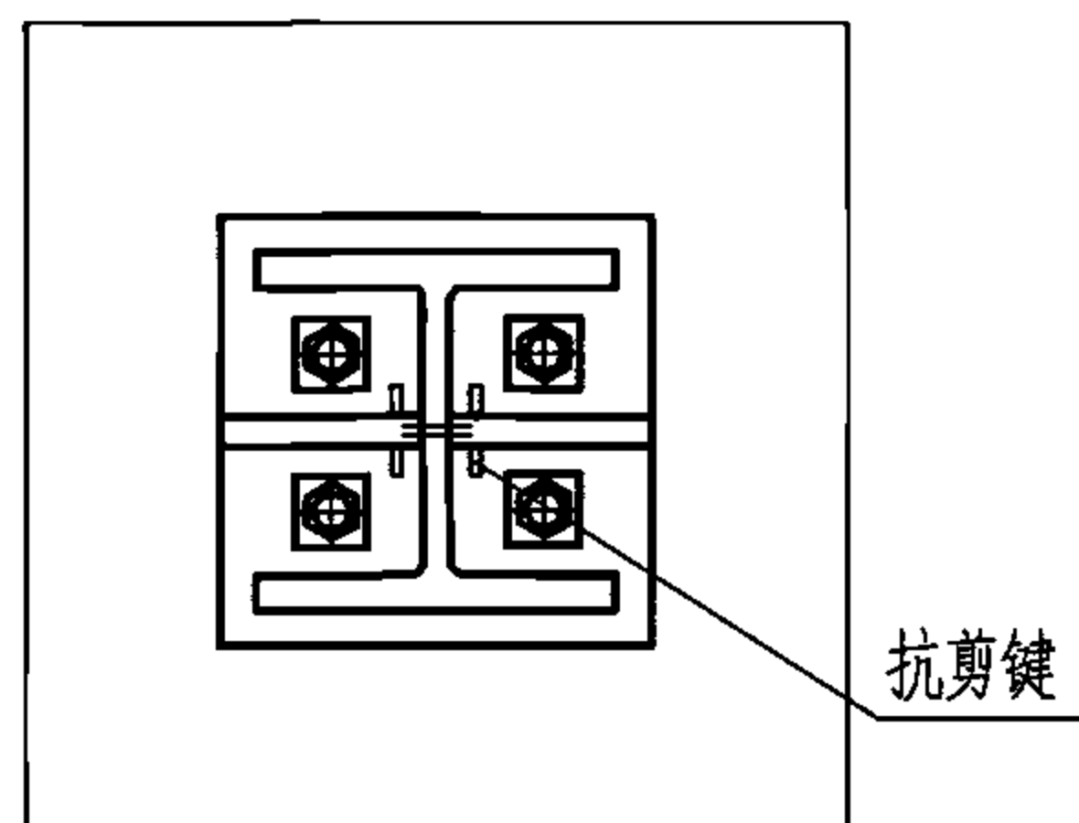
1-1
