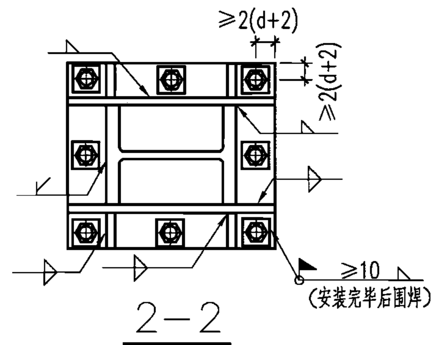
T型靴梁的板式柱脚 (柱脚b)
