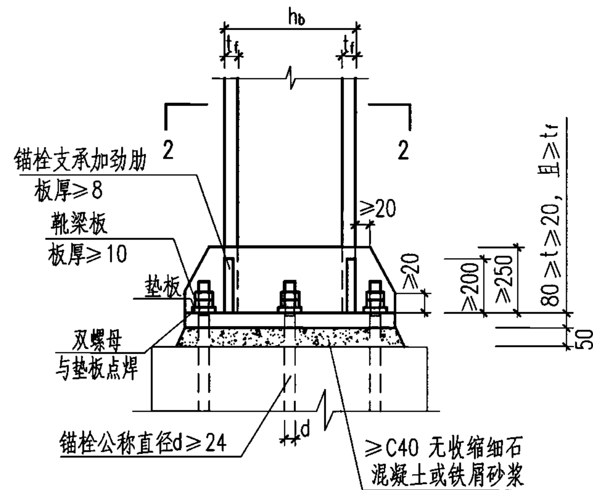
T型靴梁的板式柱脚 (柱脚b)
