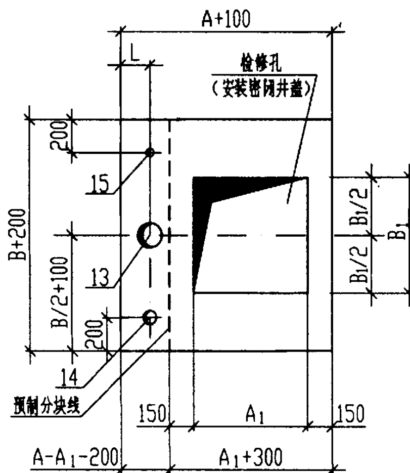
盖板留孔图
