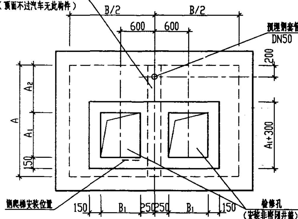
顶板留孔图
