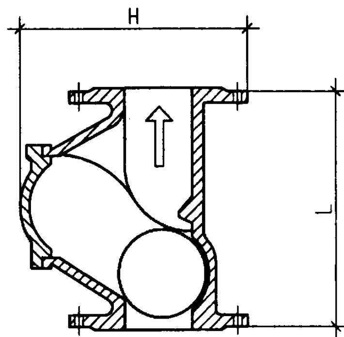
球型污水止回阀外形图
