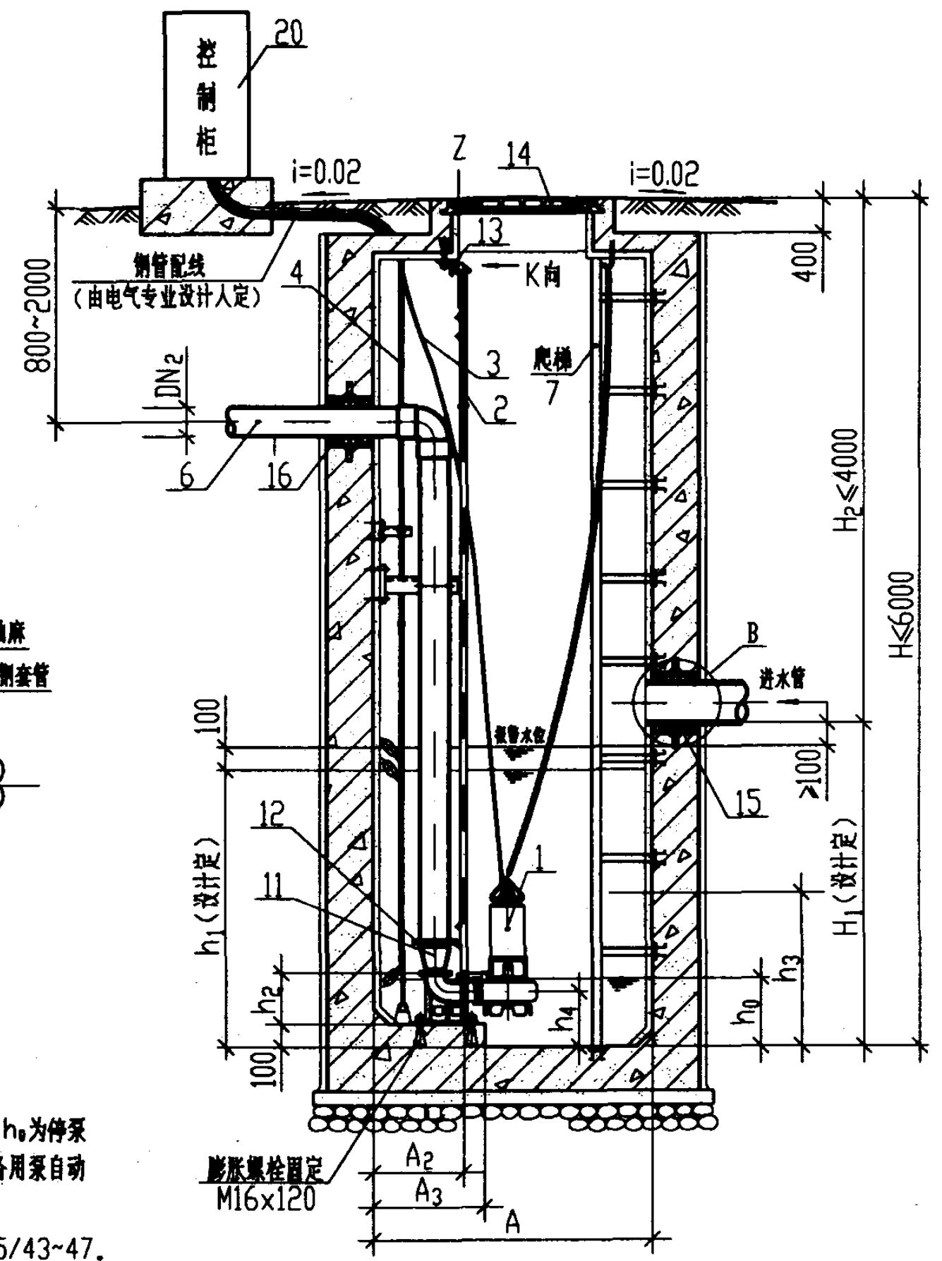
I-I剖面图
