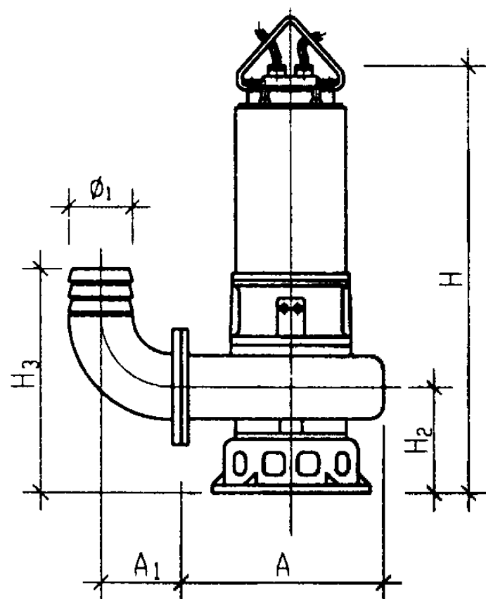
软管连接外形图
