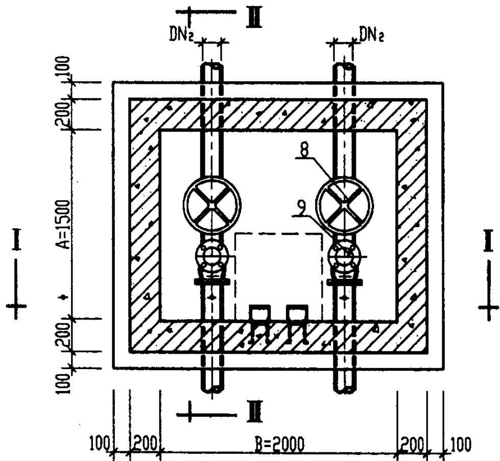
平面图
