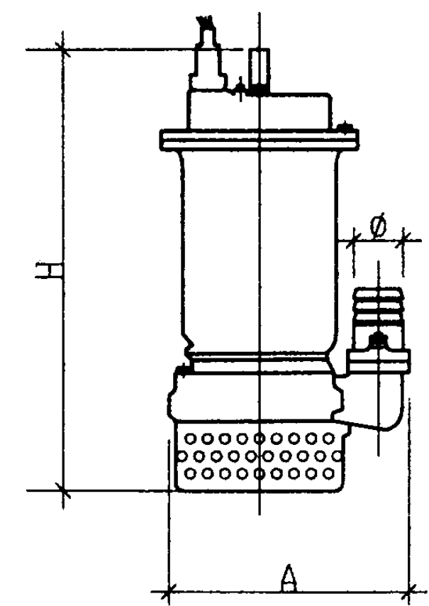
外形图
