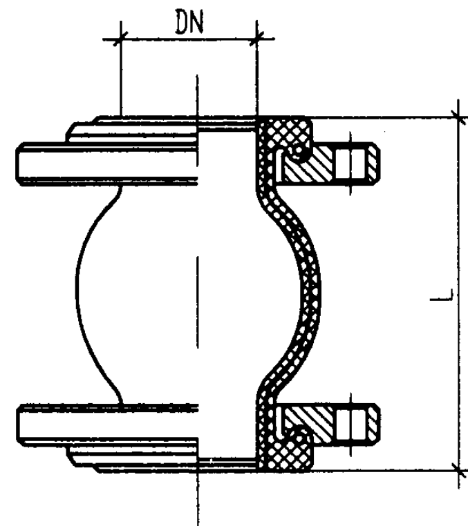
可曲挠橡胶管接头外形图
