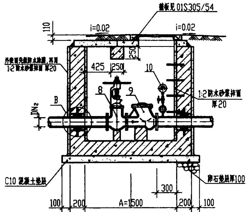
II-II 剖面图
