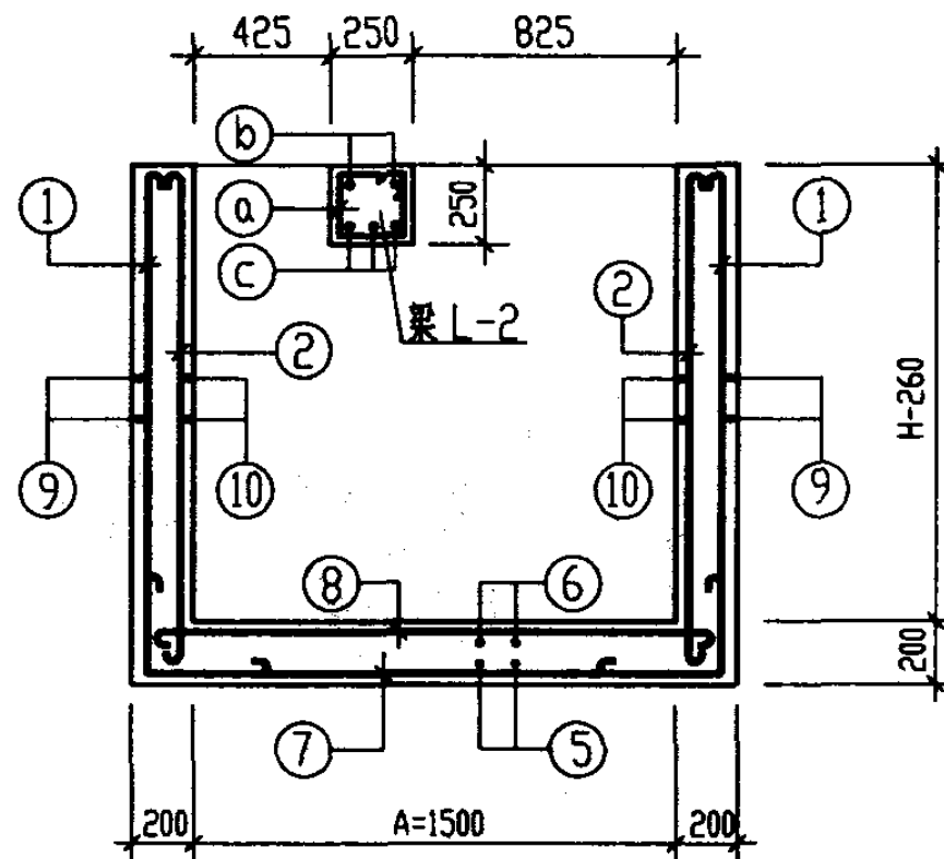
II-II 剖面图
