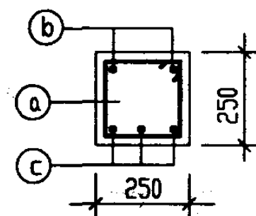
梁 L-2 剖面图
