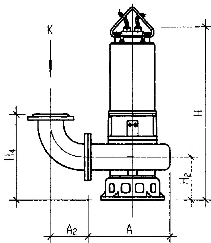
硬管连接外形图
