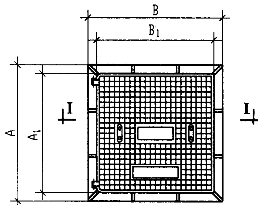
密闭井盖平面图
