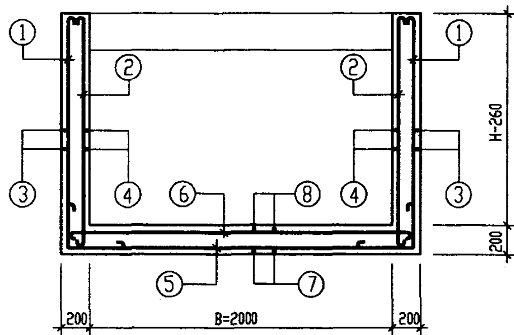
I-I 剖面图
