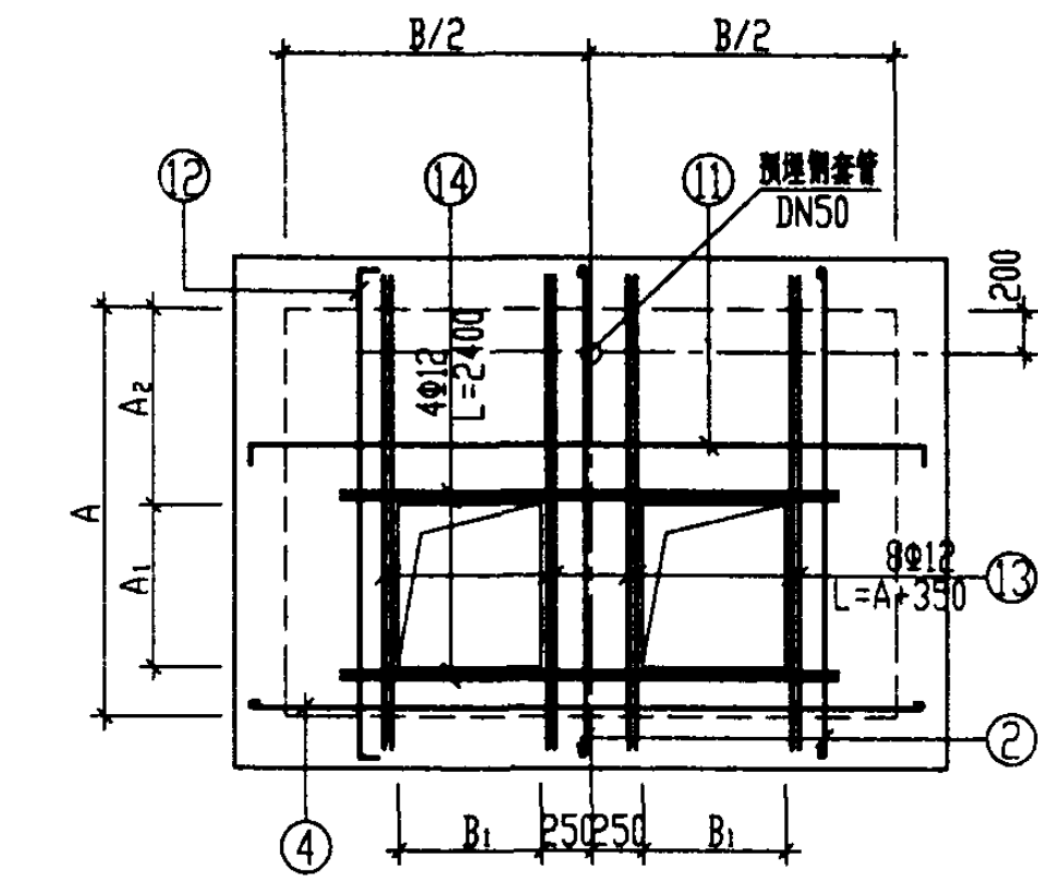
顶板配筋图 (遇洞口截断)
