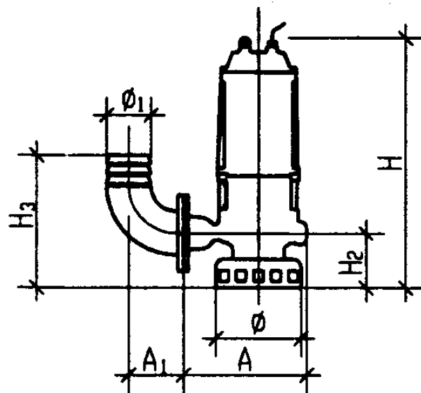
软管连接移动式安装外形图
