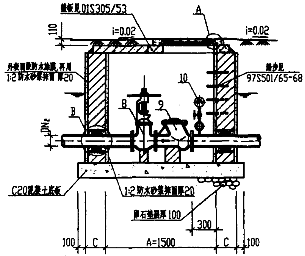
II-II 剖面图
