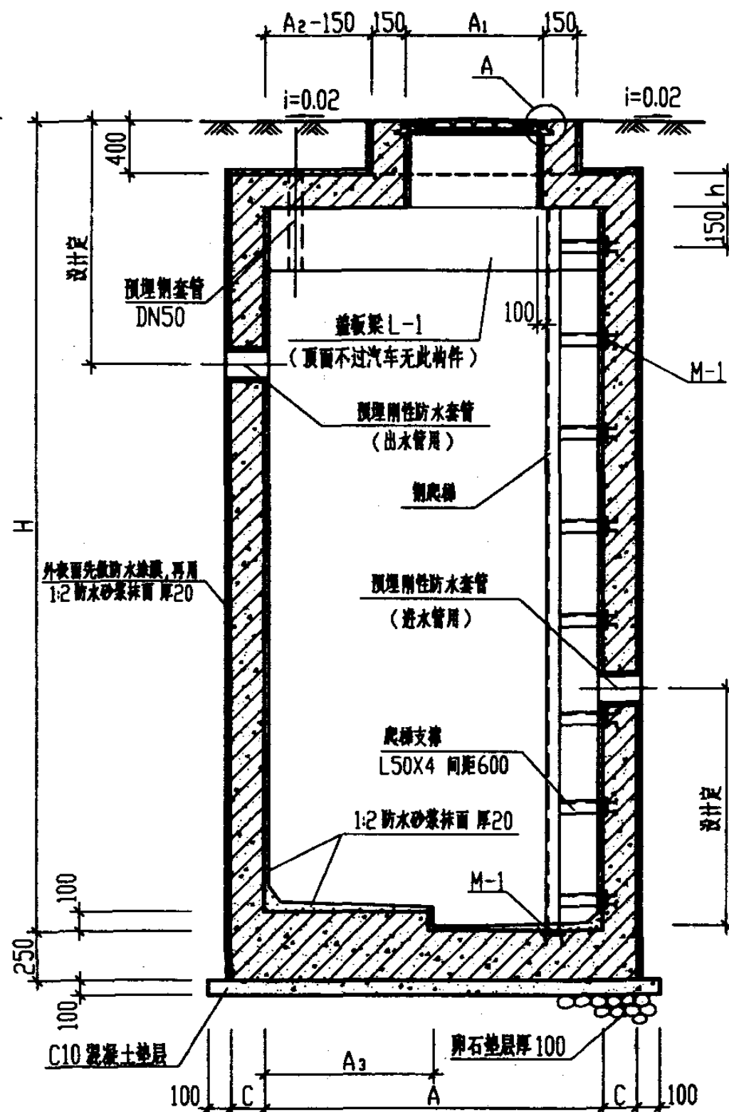
I-I 剖面图
