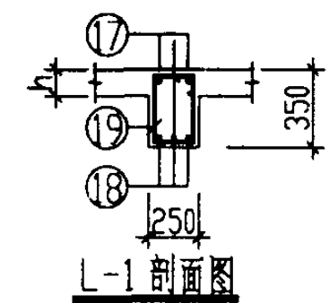
室外污水池配筋图
