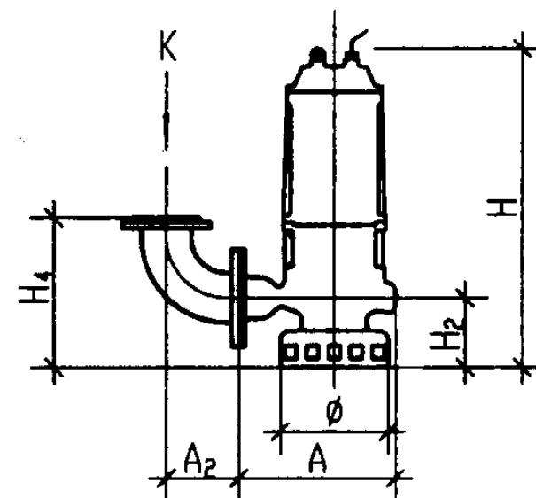
硬管连接固定式安装外形图 (K向法兰尺寸见 01S305/9)
