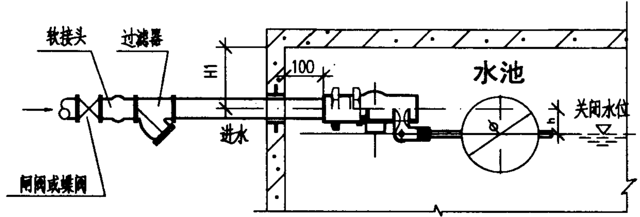
1-1 剖面图
