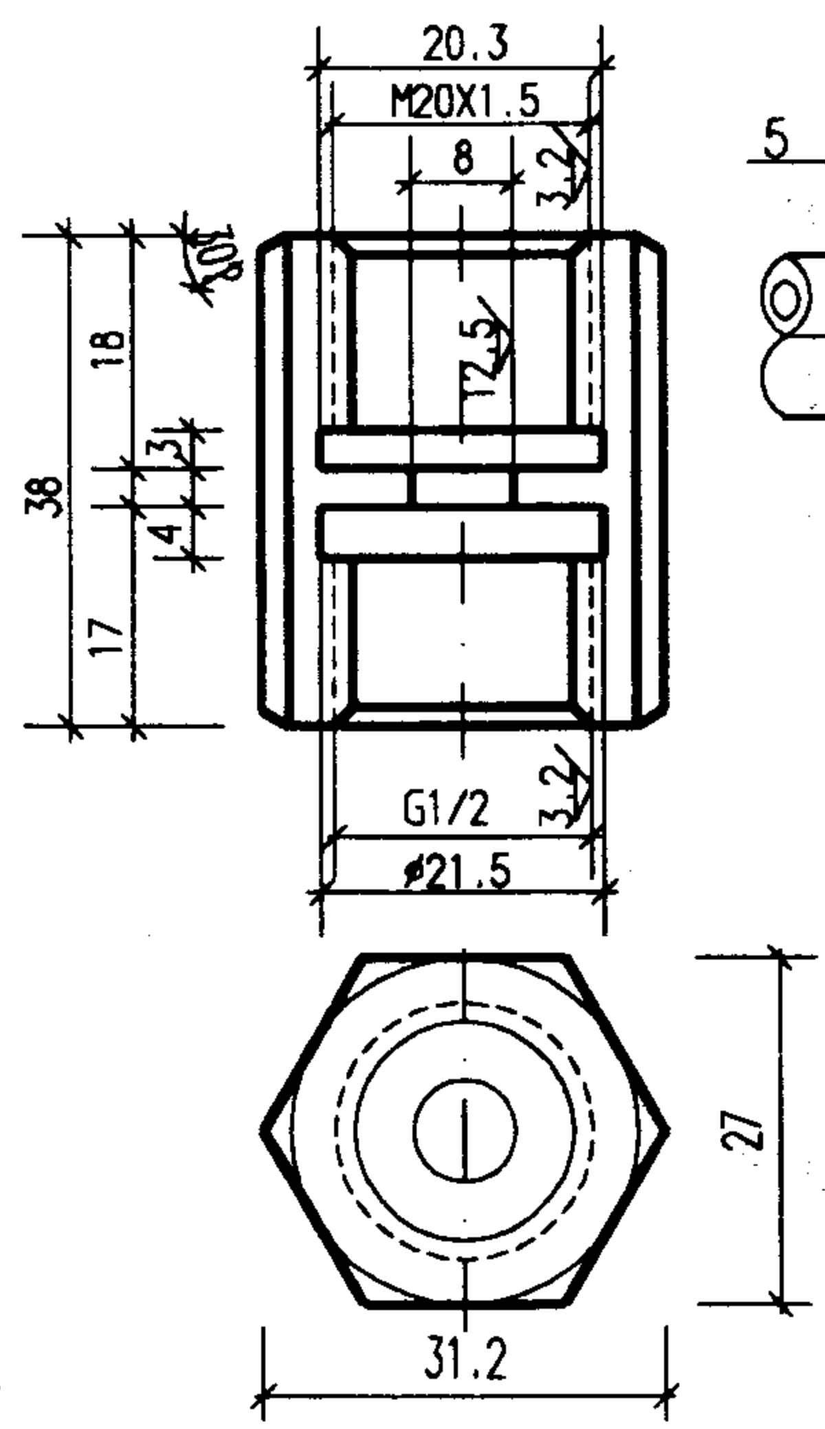
压力表接头加工图
