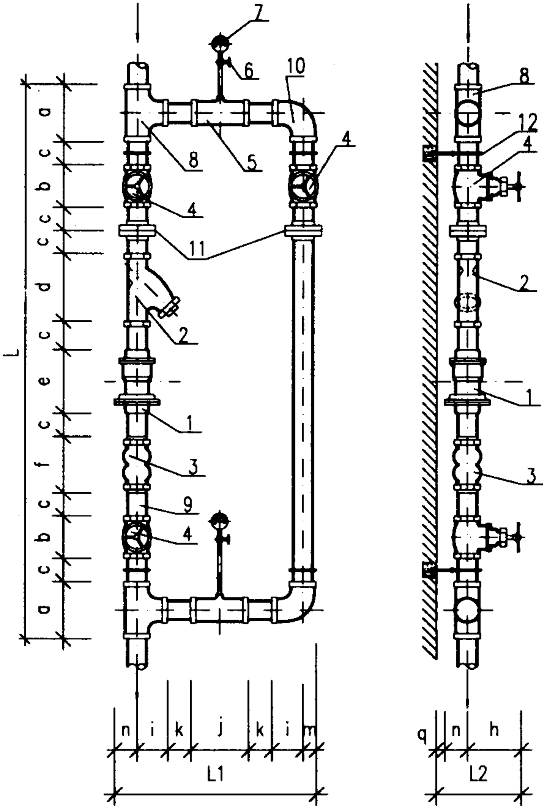
正视图
