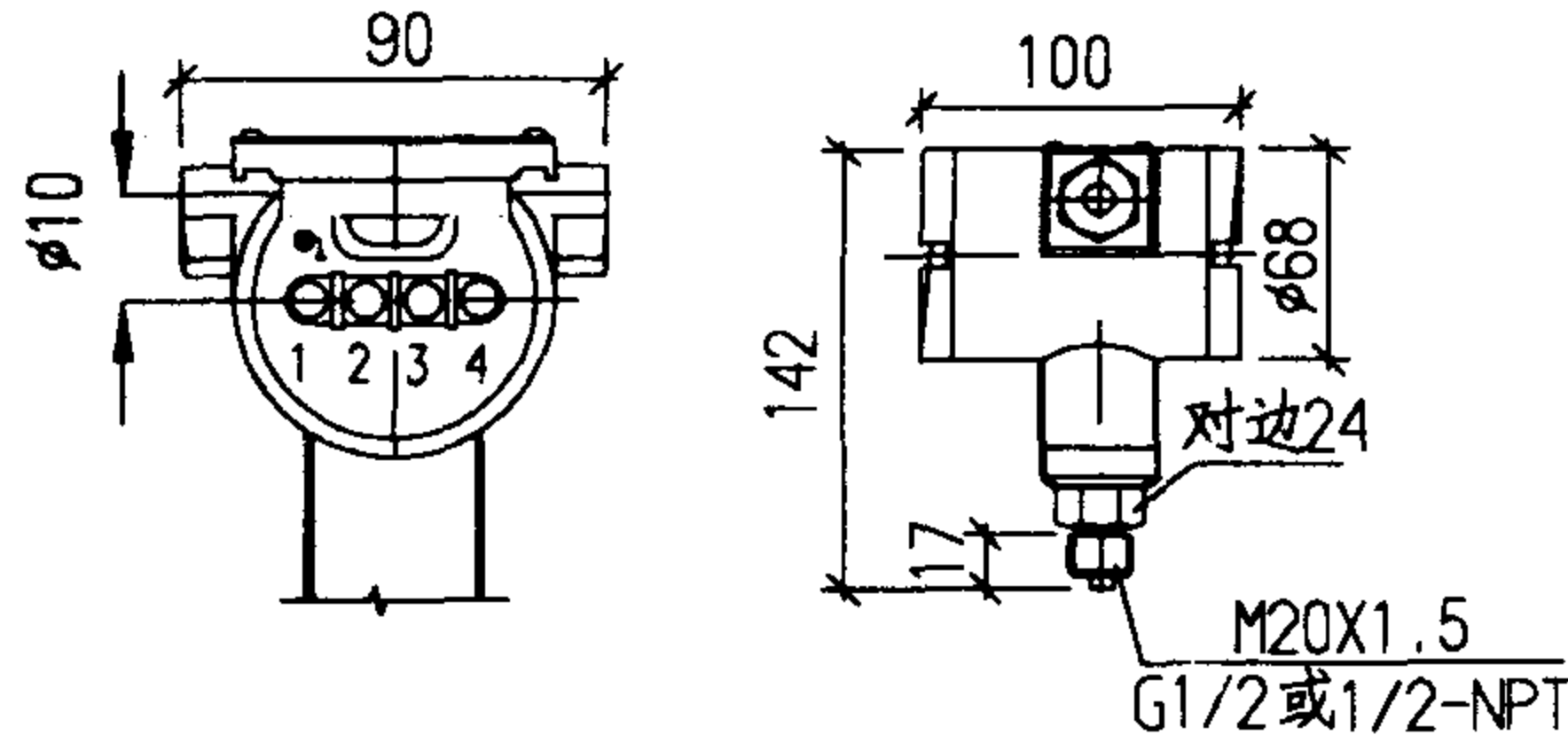
图6 压力变送器外型图
