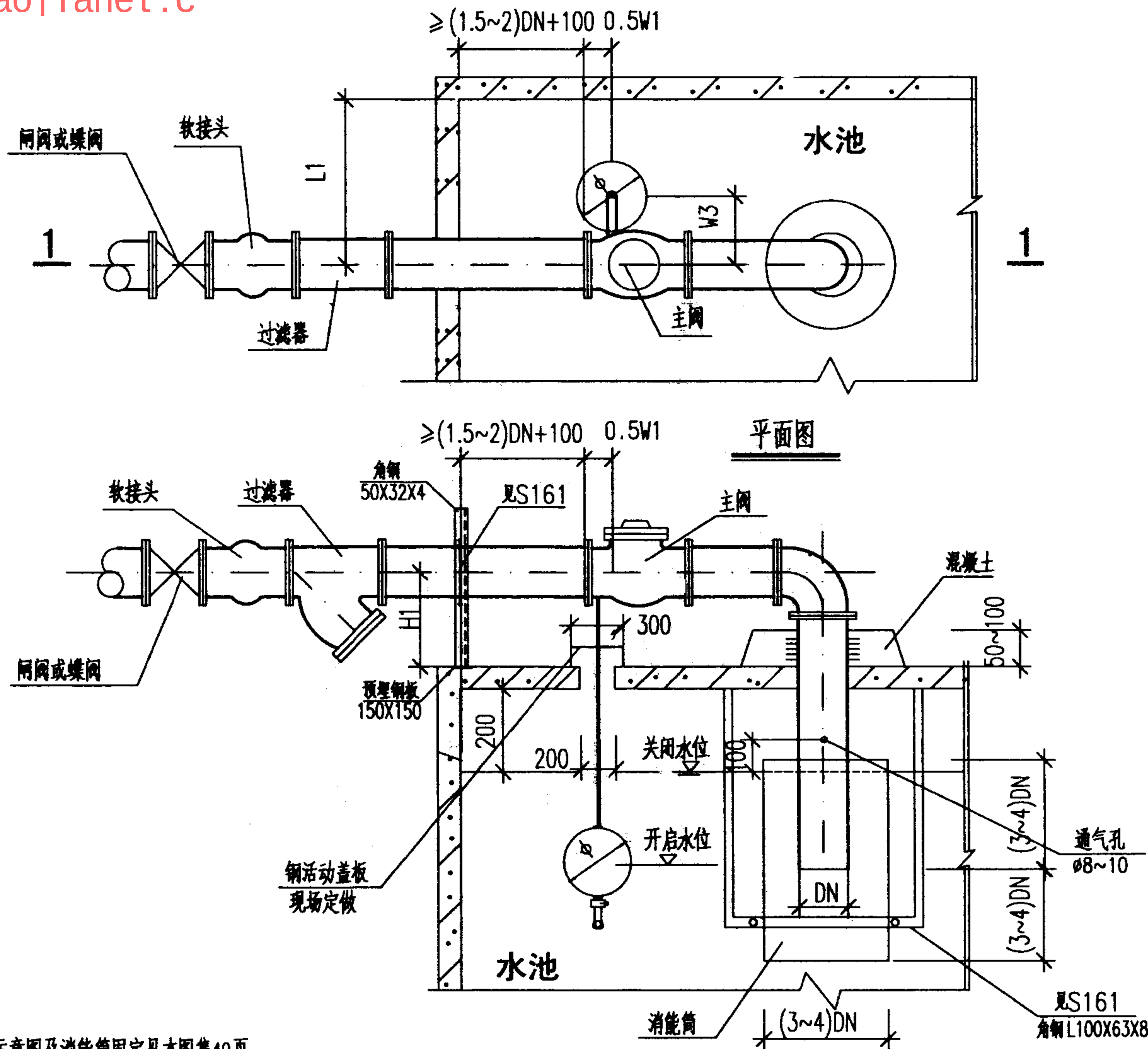
1-1 剖面图
