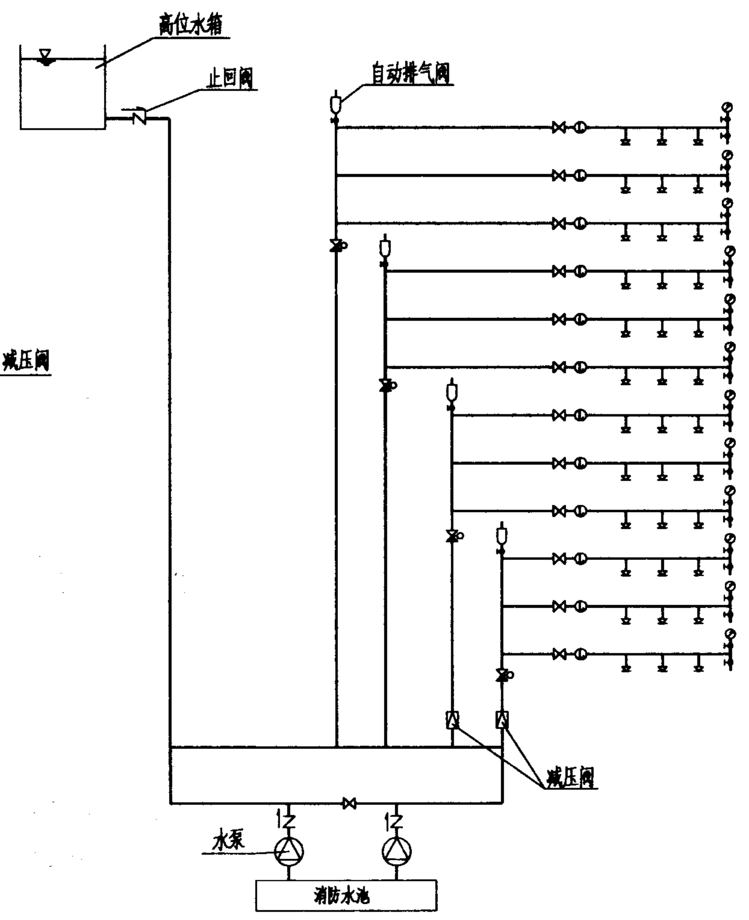
减压阀自动喷水灭火供水方式
