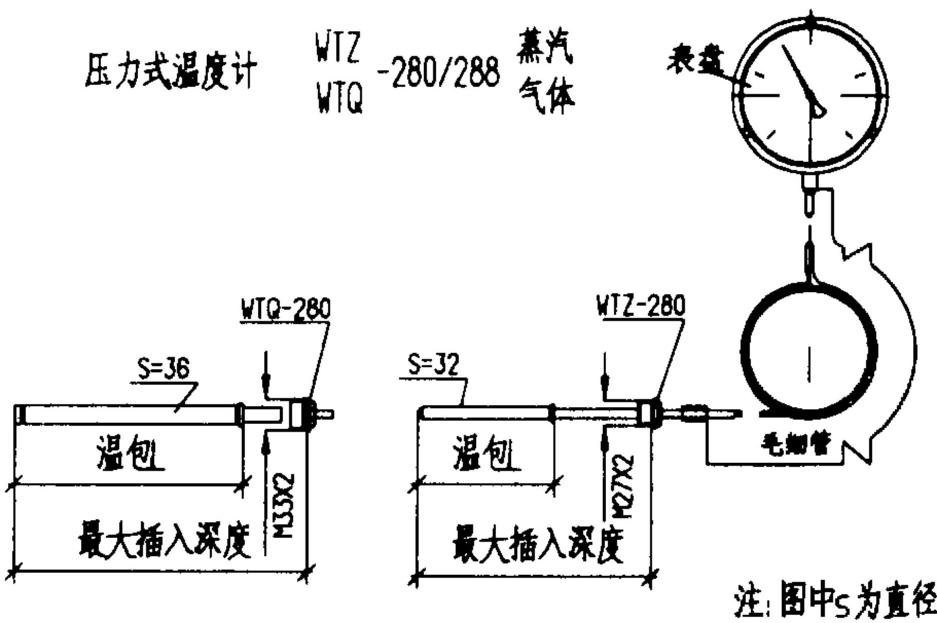
图1 压力式温度计外型图
