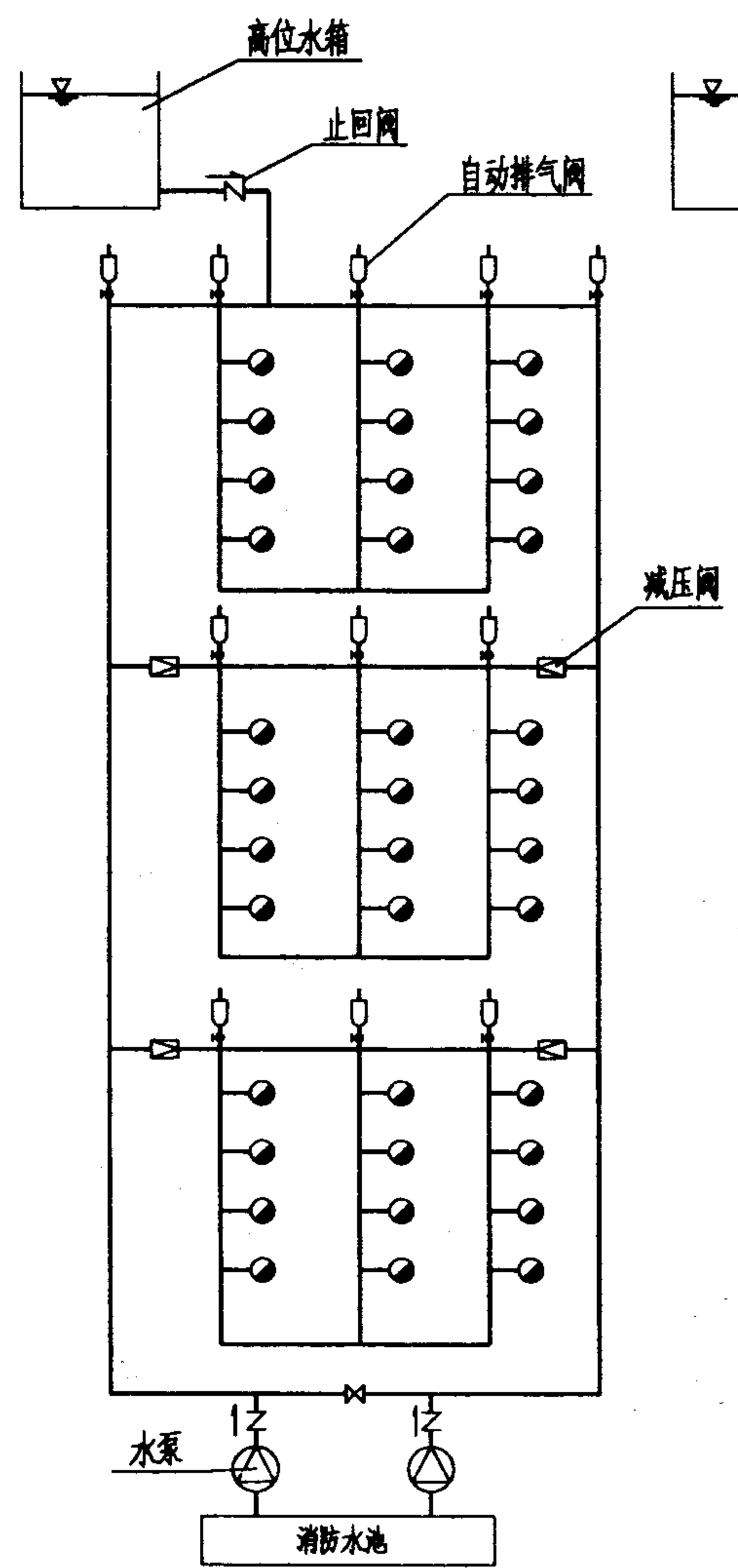
减压阀并联消火栓供水方式
