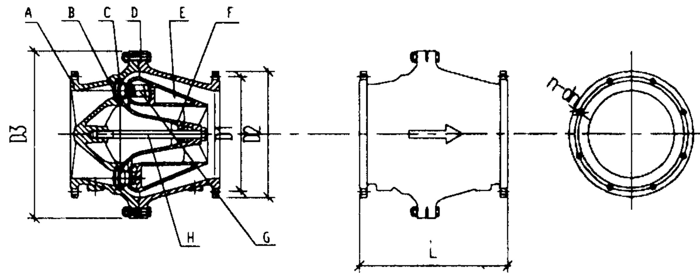
图4 冠龙DRVZ型静音止回阀结构图
