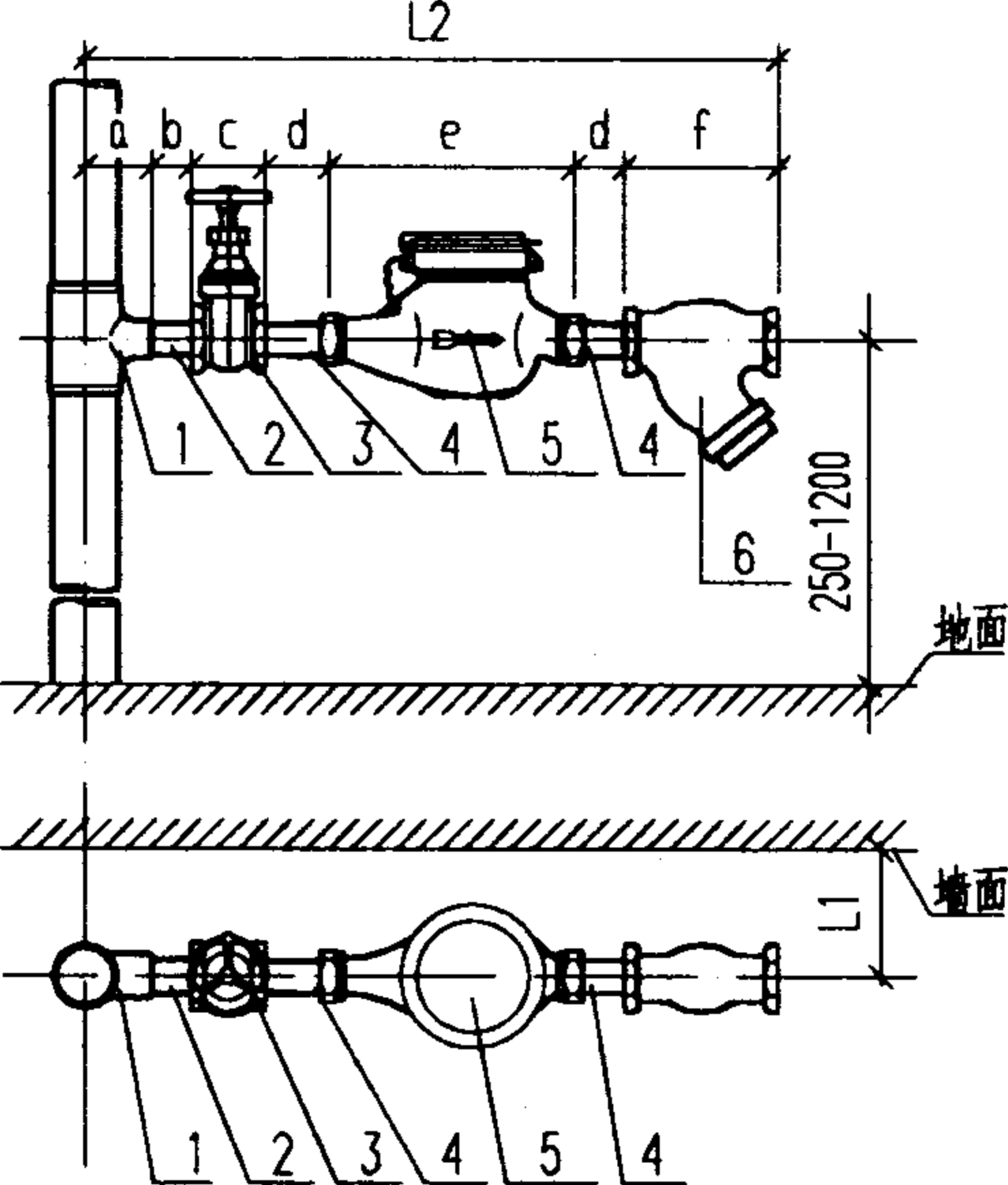
乙型安装图
