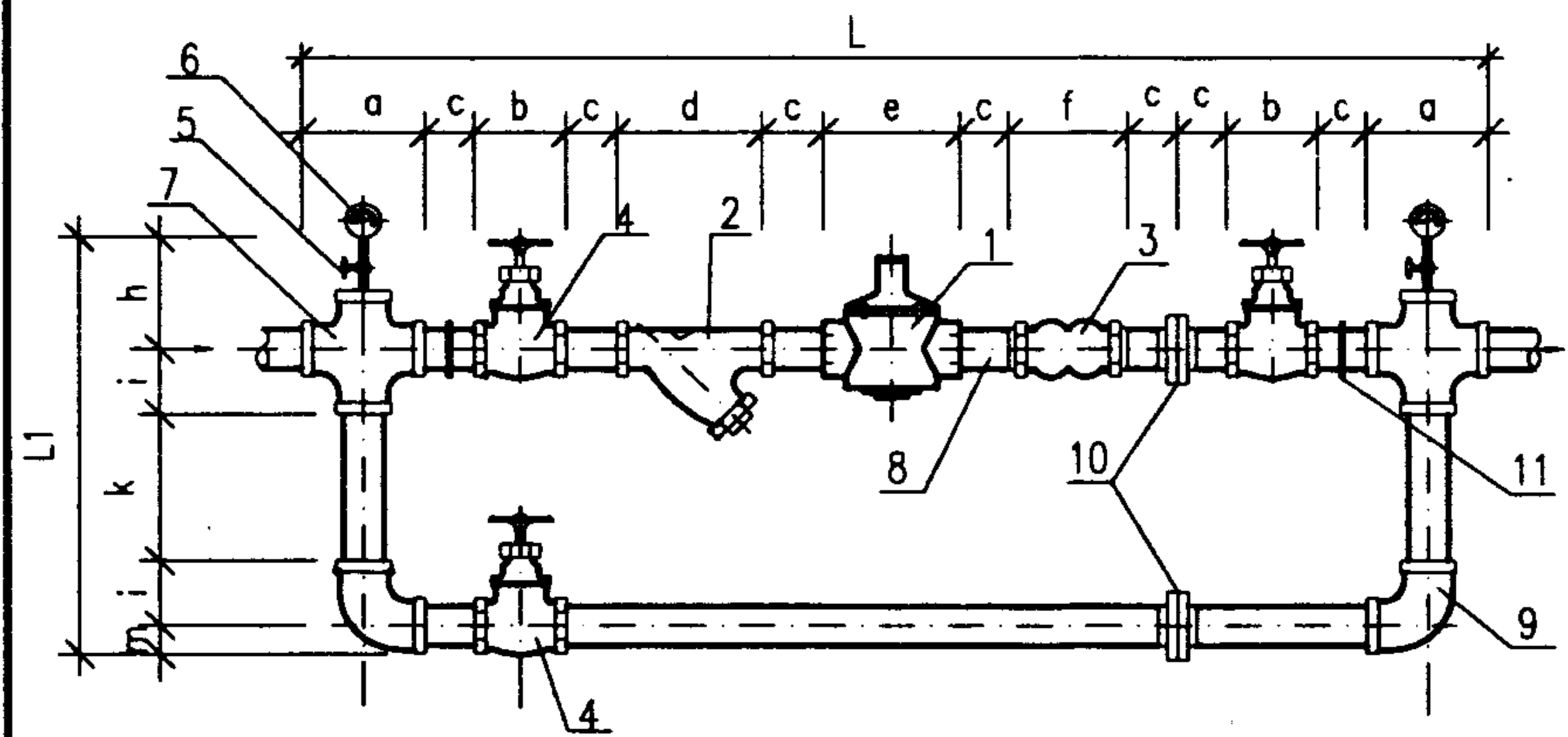
正视图
