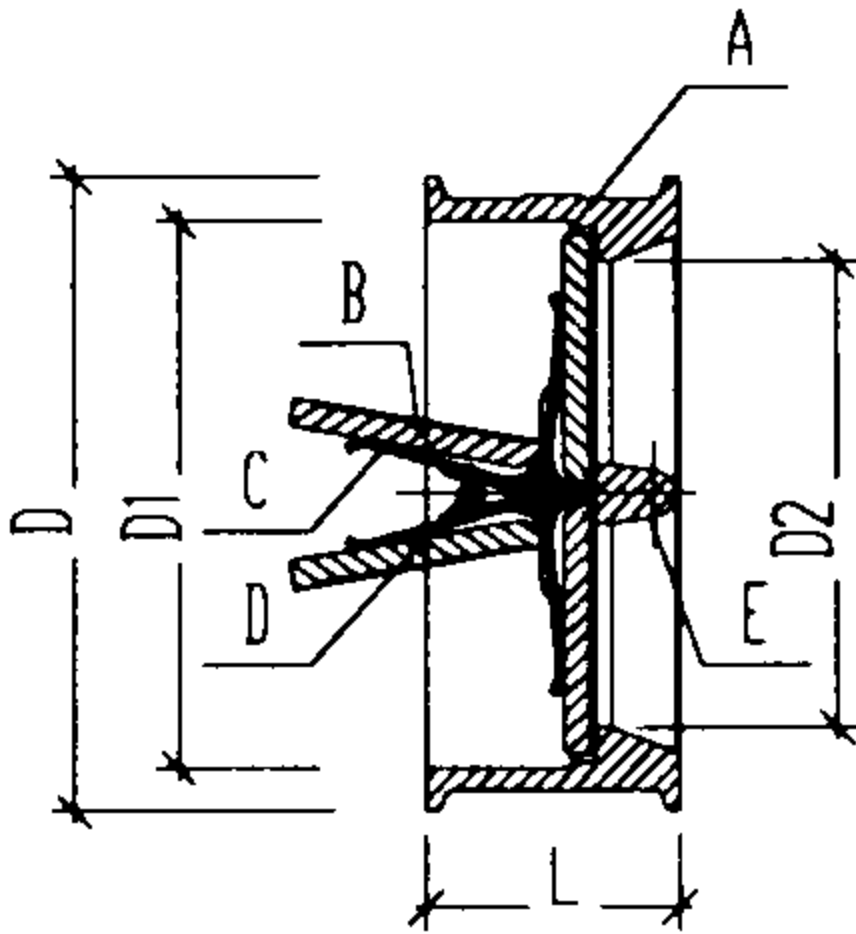
图2 冠龙DDCV型双瓣止回阀
