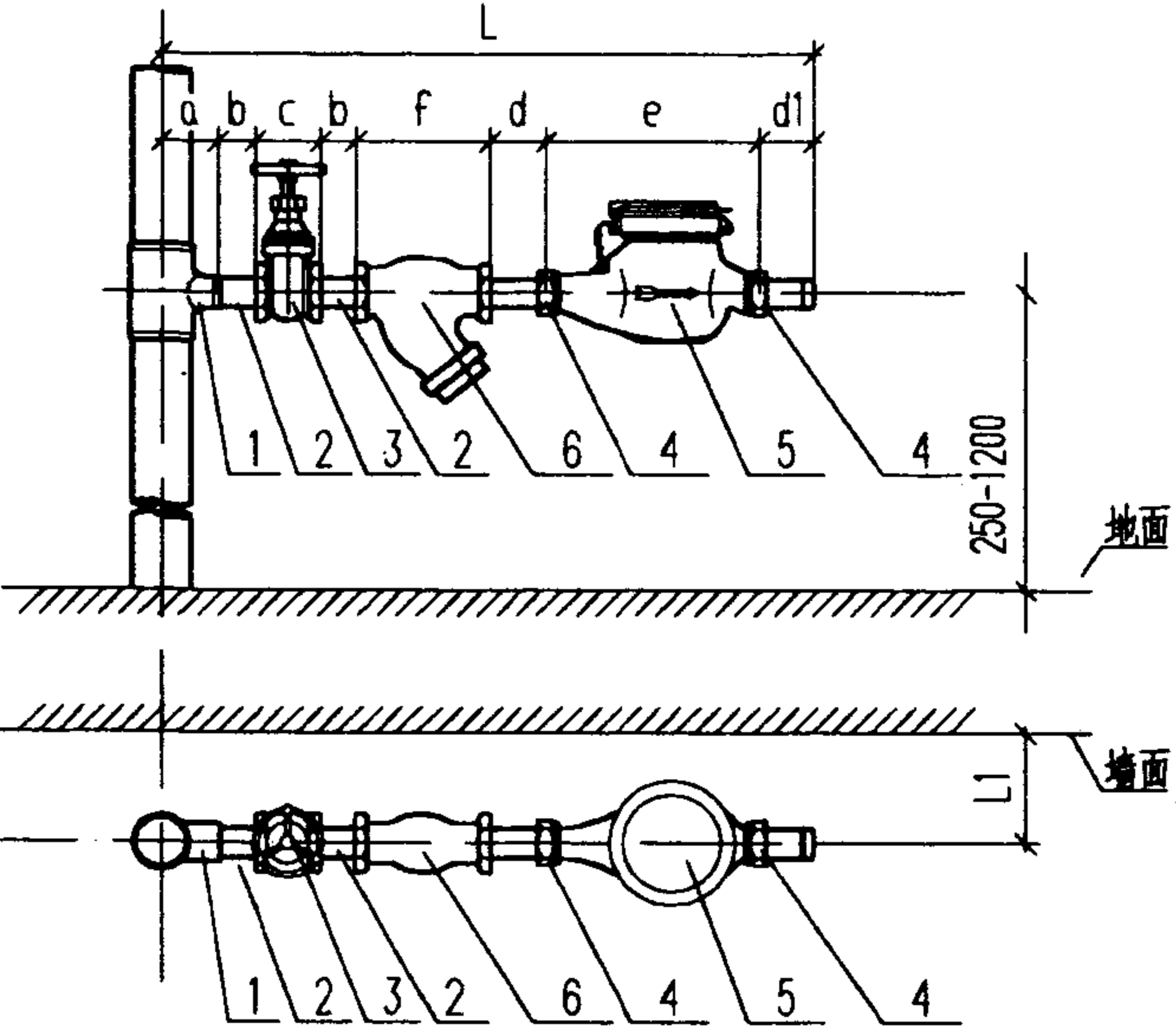
甲型安装图
