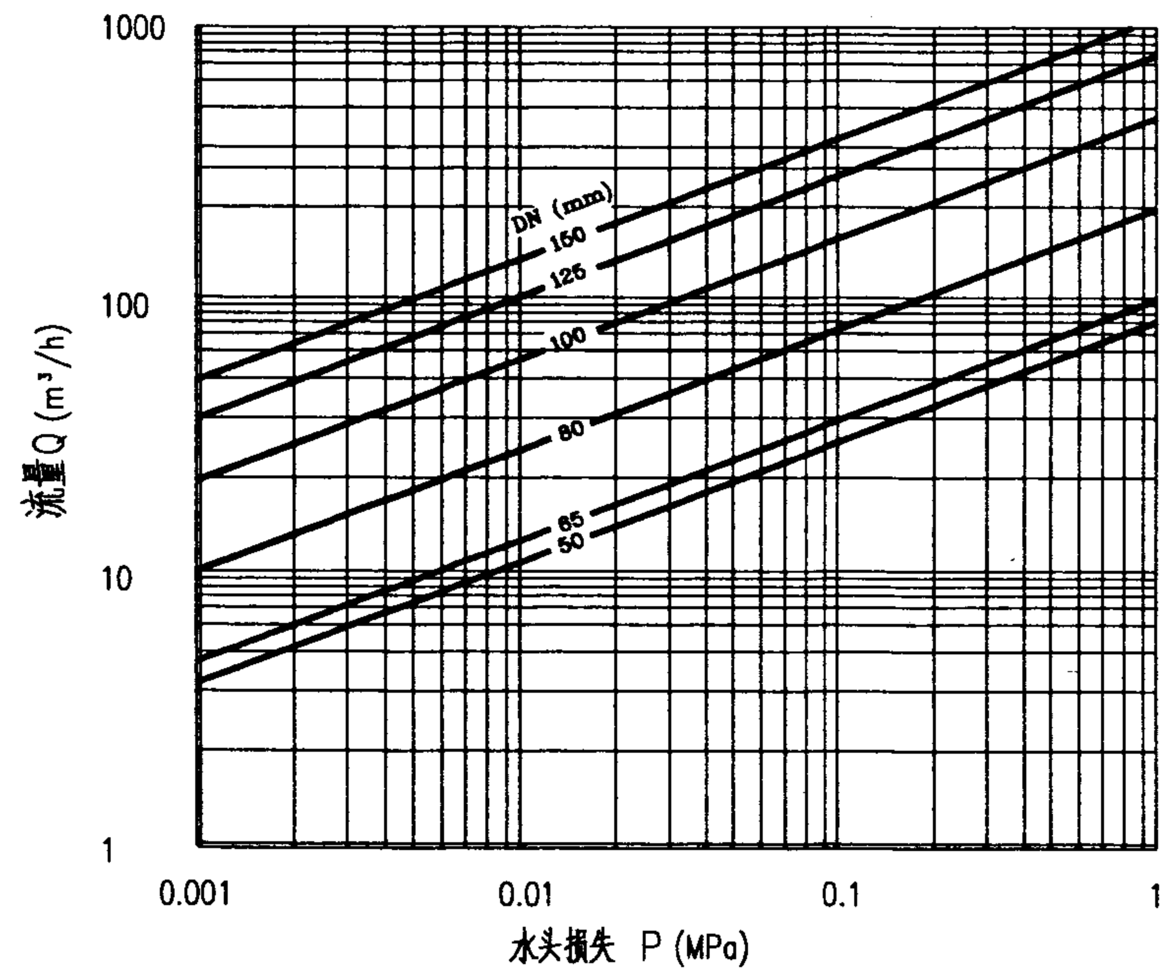
YW减压阀流量水头损失特性曲线
