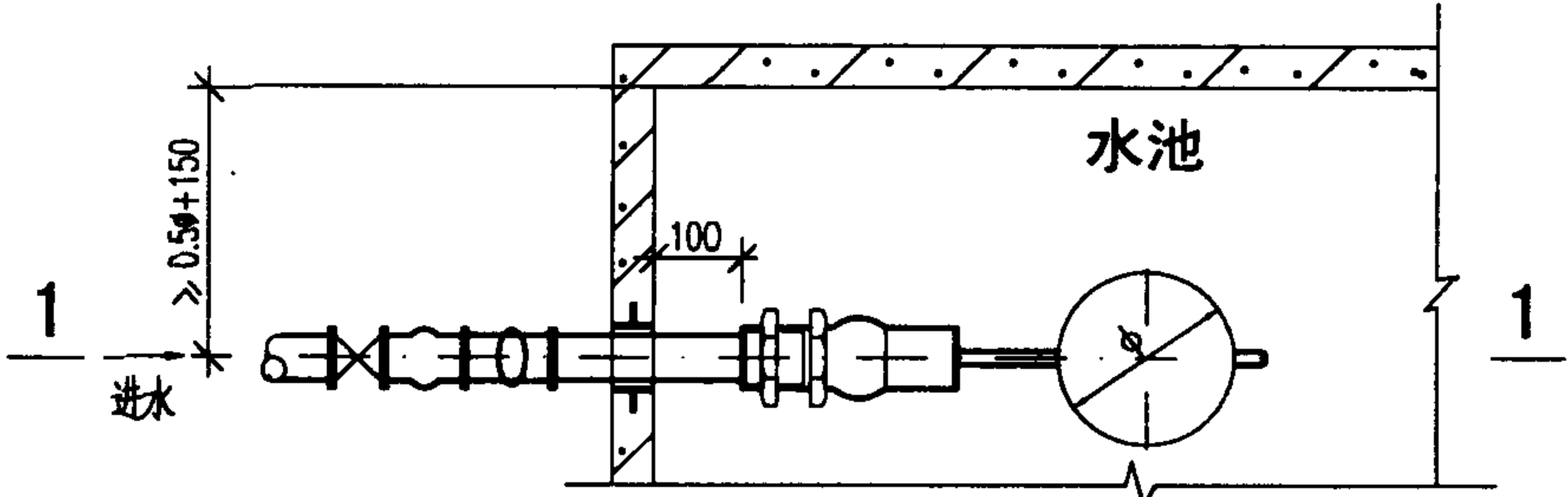
平面图
