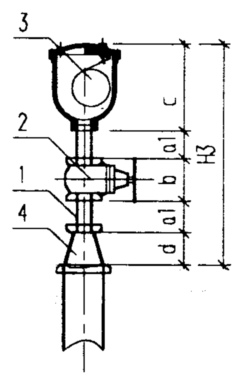
ARSX微量排气阀乙型安装
