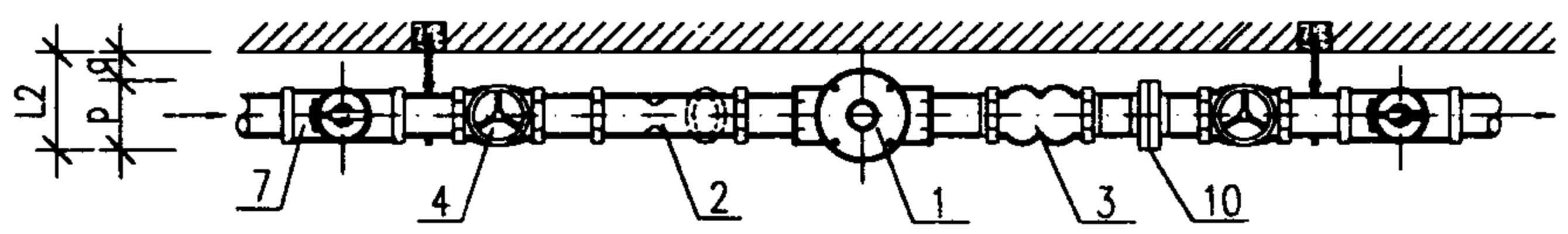
俯视图
