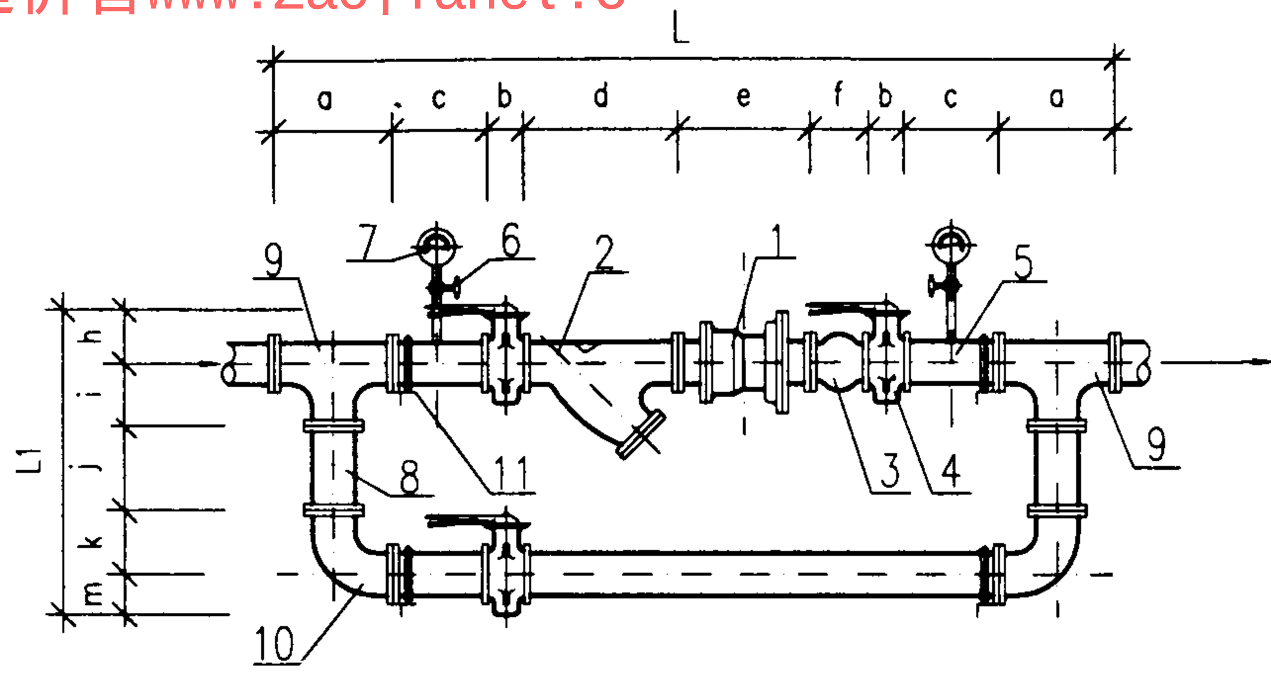
正视图
