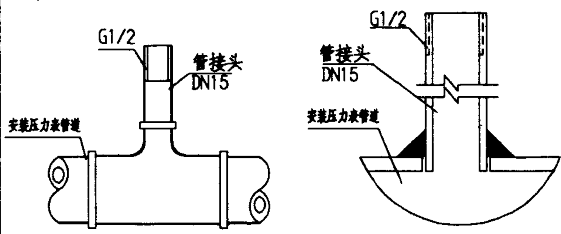
管接头A型
