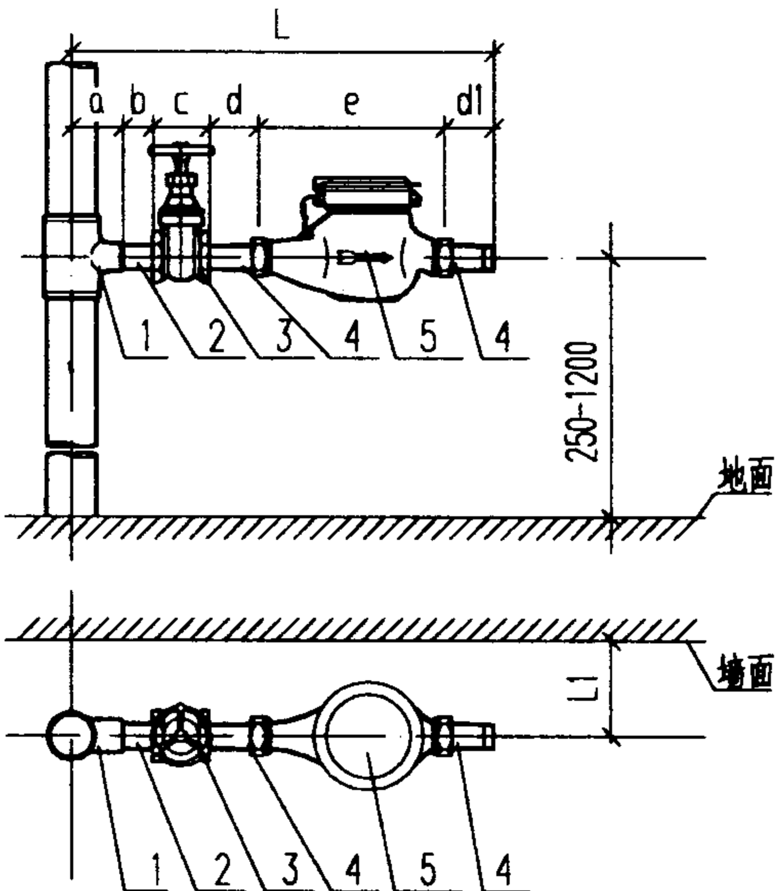
丙型安装图
