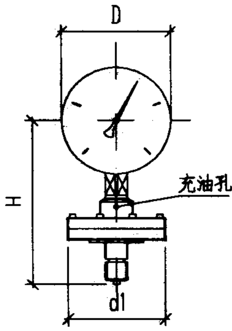
图3 隔膜压力表外型图
