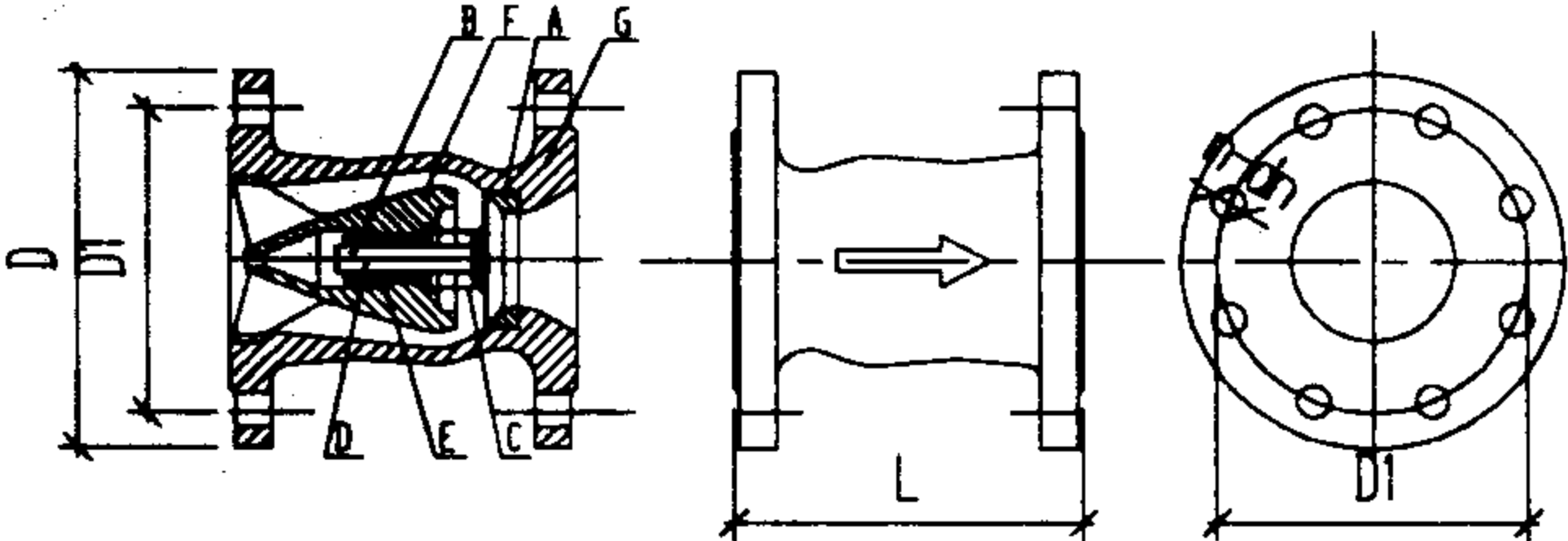
图3 冠龙DRVZ型静音止回阀结构图
