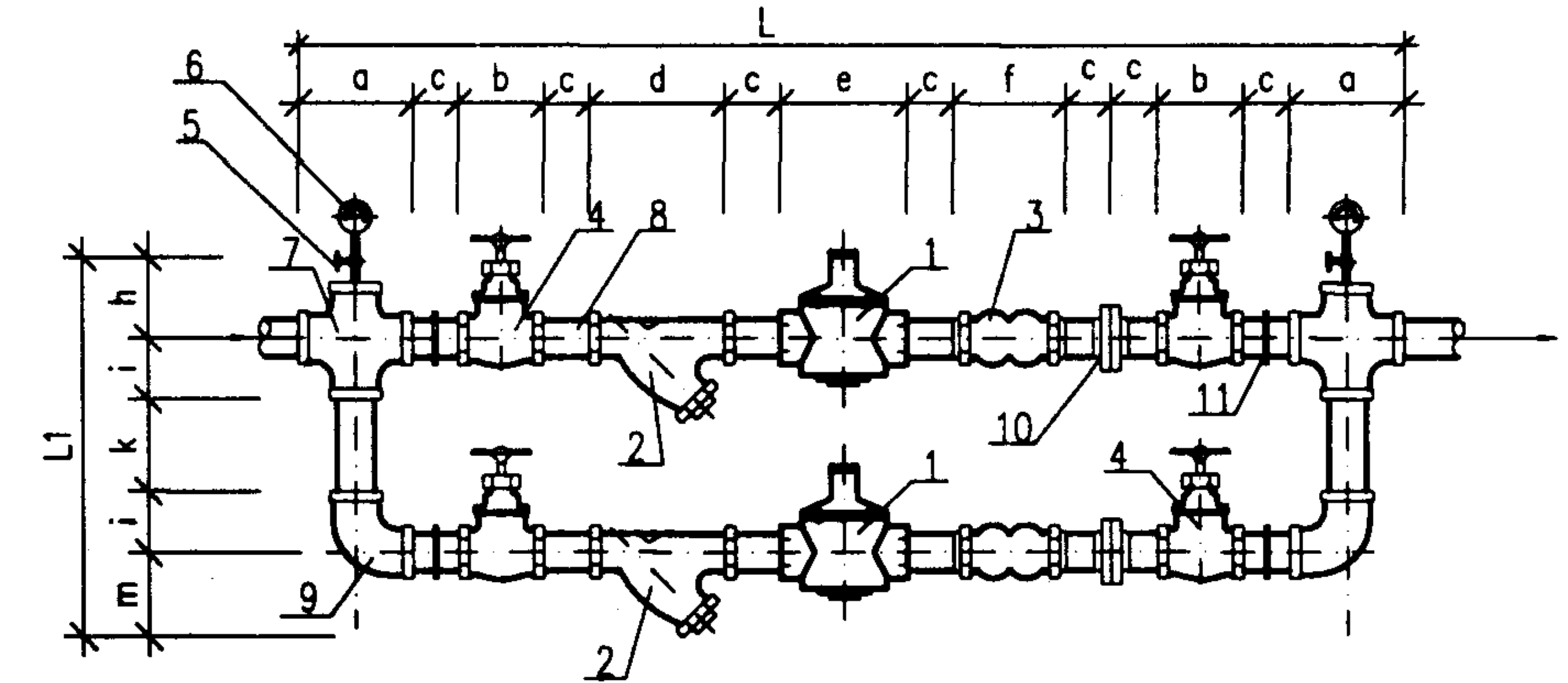
正视图
