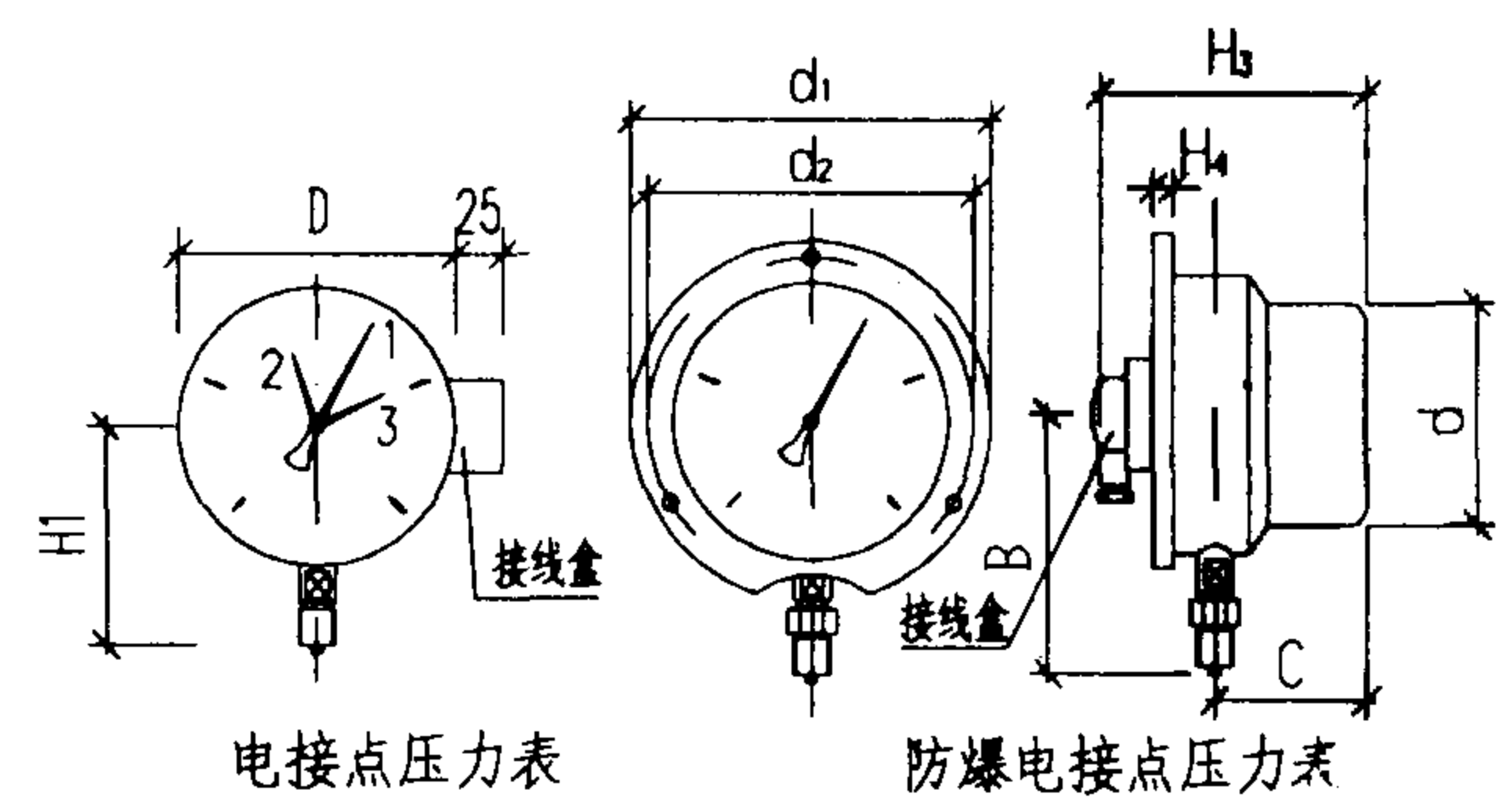
图4 电接点压力表外型图
