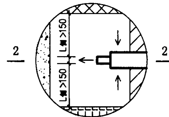
给排气风帽排气出口安全间距示意图 (水平向前排气) (万和公司)
