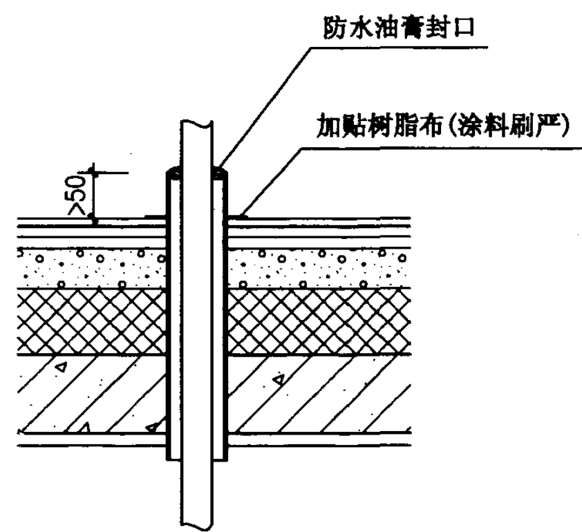
套管穿平屋面节点
