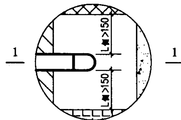
风帽排气出口安全间距示意图
