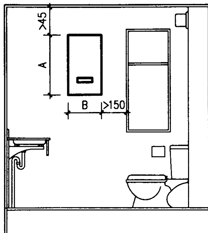
立面图
