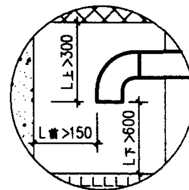
1-1剖面
