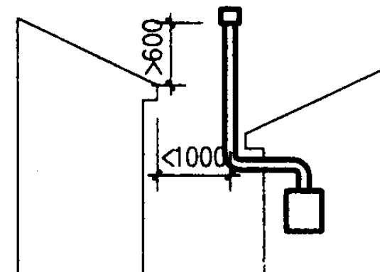
风帽高出屋檐距离示意图
