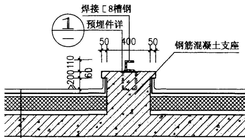
平屋面支座安装节点(一)
