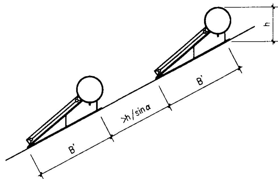
坡屋面坡面安装
