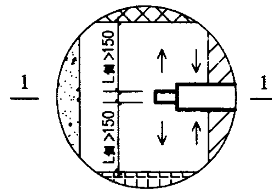
给排气风帽排气出口安全间距示意图 (垂直360° 排气) (三益公司)
