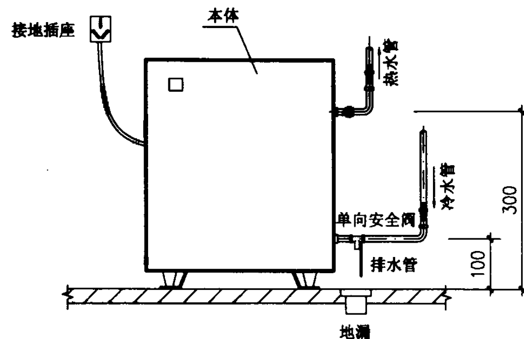
安装详图
