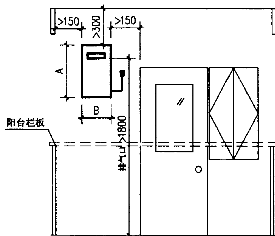
立面图
