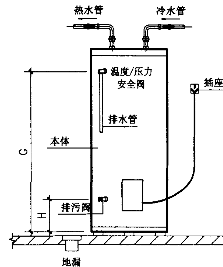
上方出水安装详图
