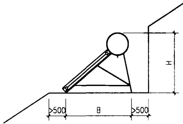
坡屋面嵌入安装
