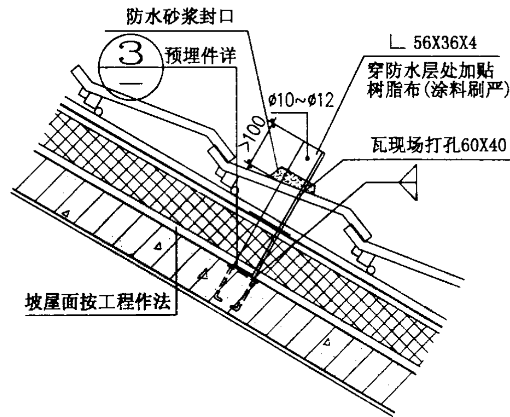
坡屋面支座安装节点(一)
