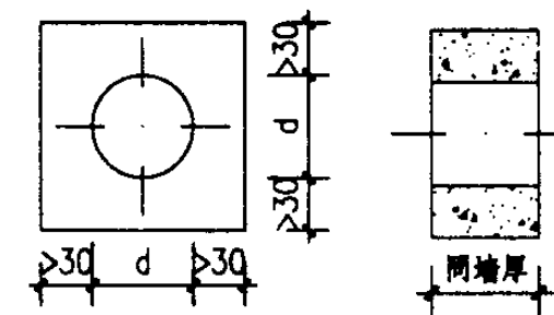
预制带洞混凝土块
