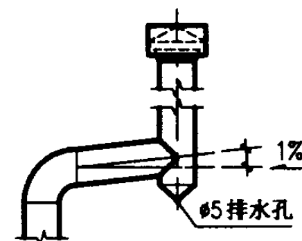
圆型防风帽
