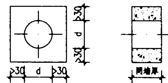
预制带洞混凝土块
