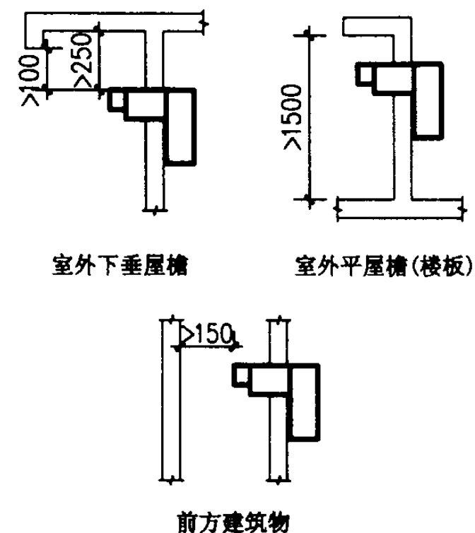
给排气风帽的周边条件示意图(剖面)
