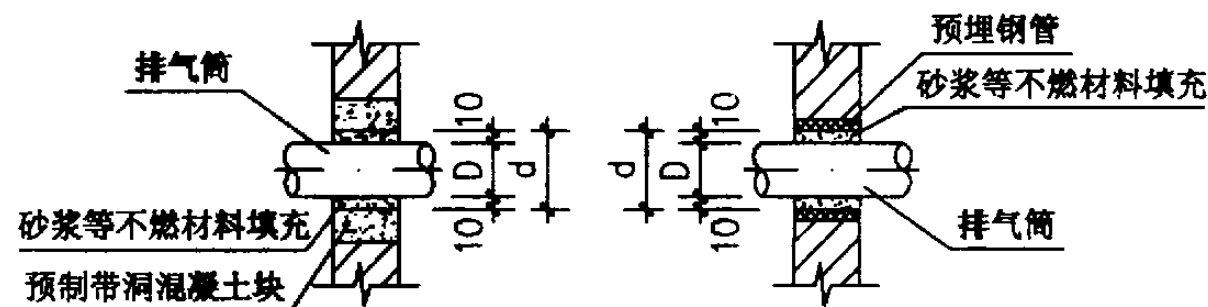
节点A
