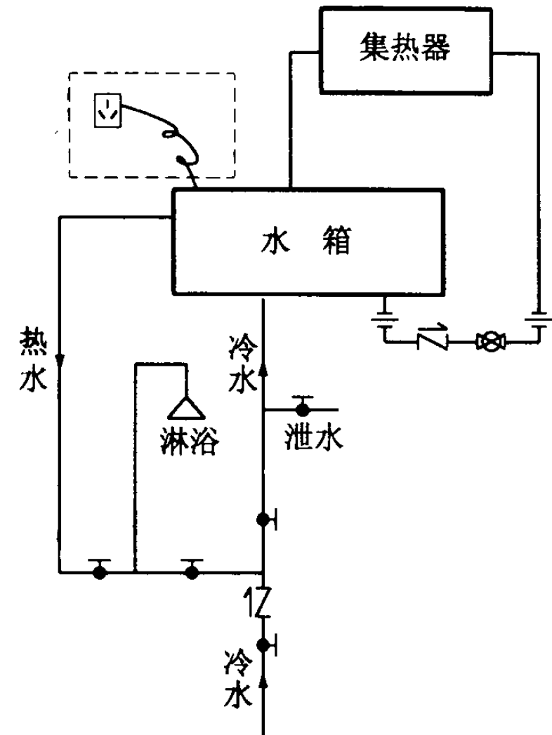
分离式顶水法原理图
