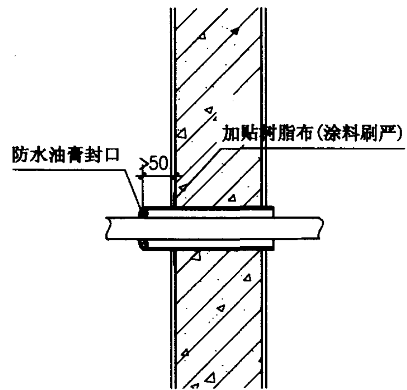
套管穿墙节点
