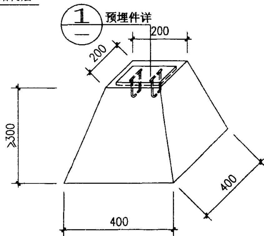
平屋面支座安装节点(二)
