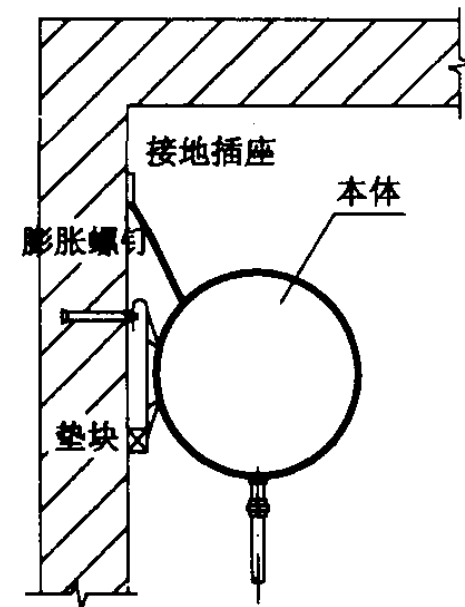
侧面图 (详)
