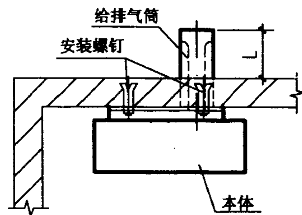
平面图
