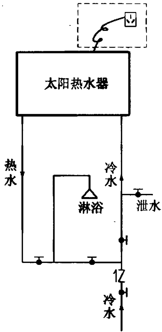
紧凑式顶水法原理图
