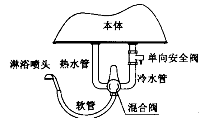
出口敞开式
