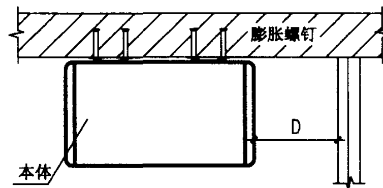
平面图 (详)
