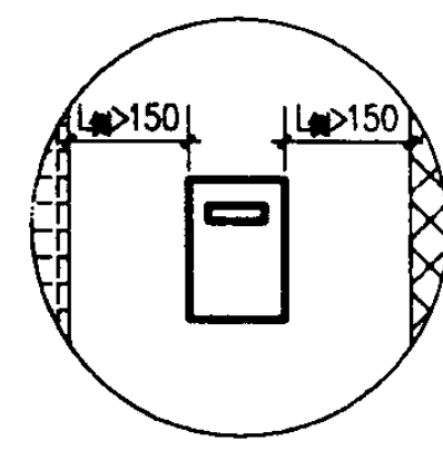
排气出口与周围建筑物的间距
