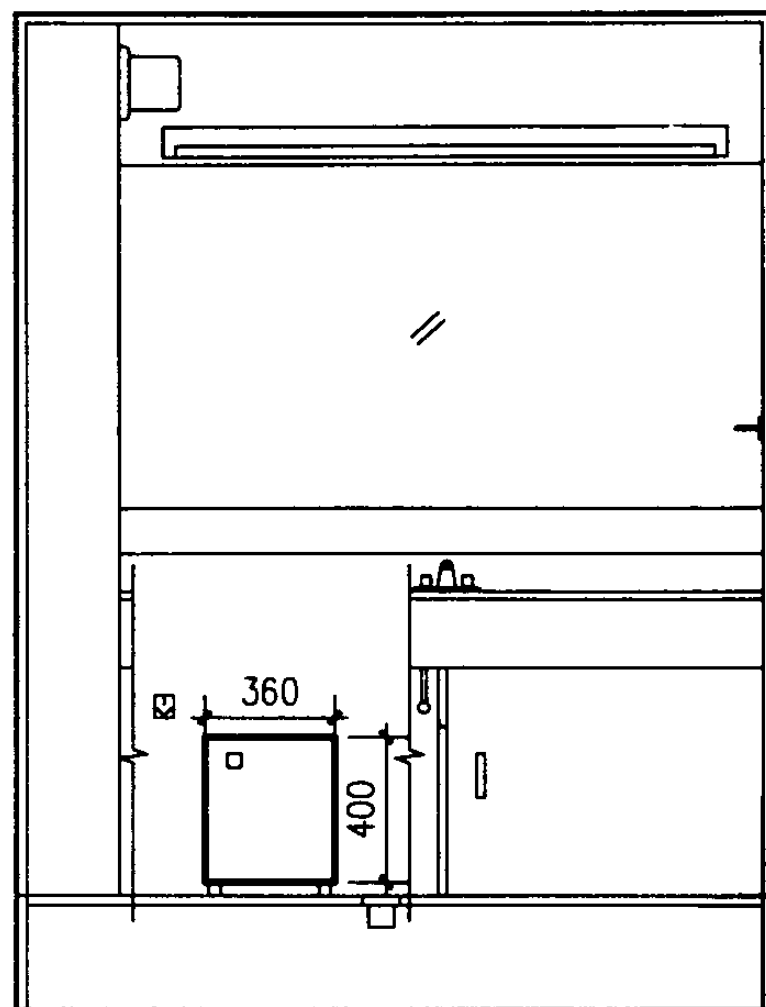
立面图
