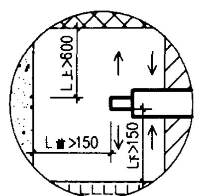
1-1剖面
