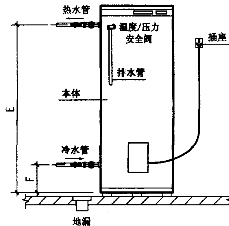
侧方出水安装详图
