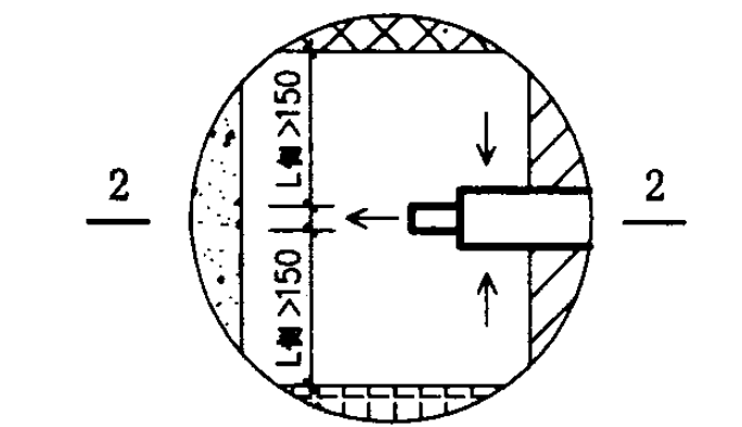
给排气风帽排气出口安全间距示意图 (水平向前排气) (万和公司)
