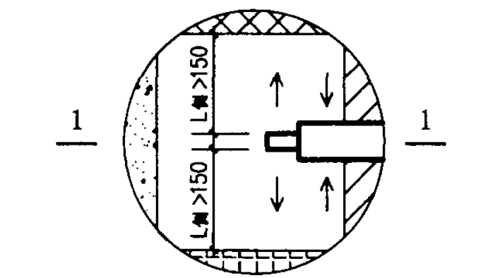
给排气风帽排气出口安全间距示意图 (垂直360° 排气) (三益公司)
