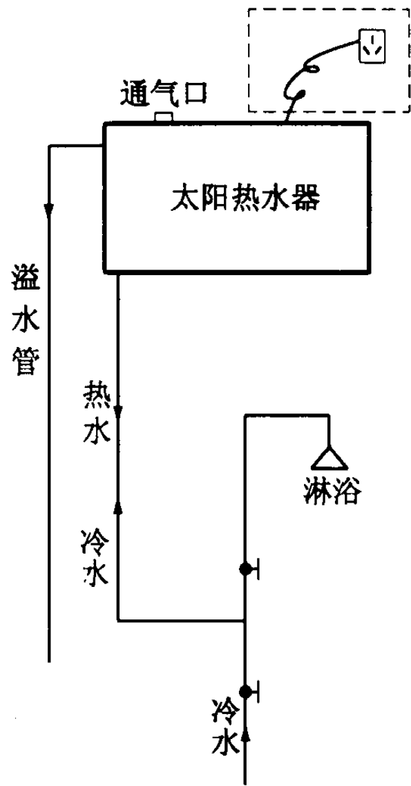
紧凑式落水法原理图
