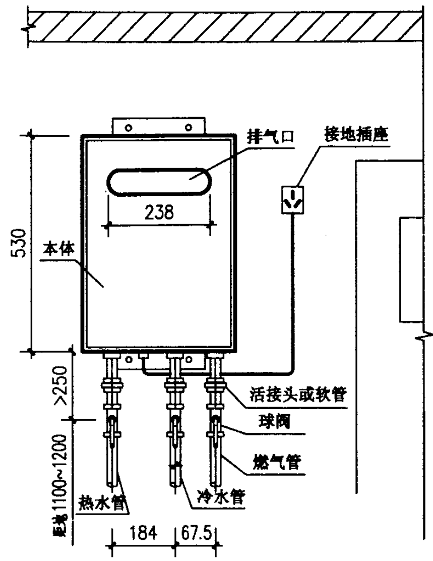
立面图
