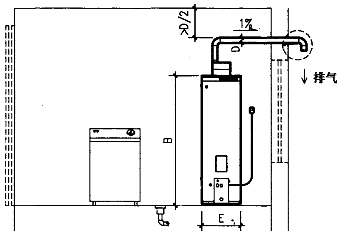
立面图
