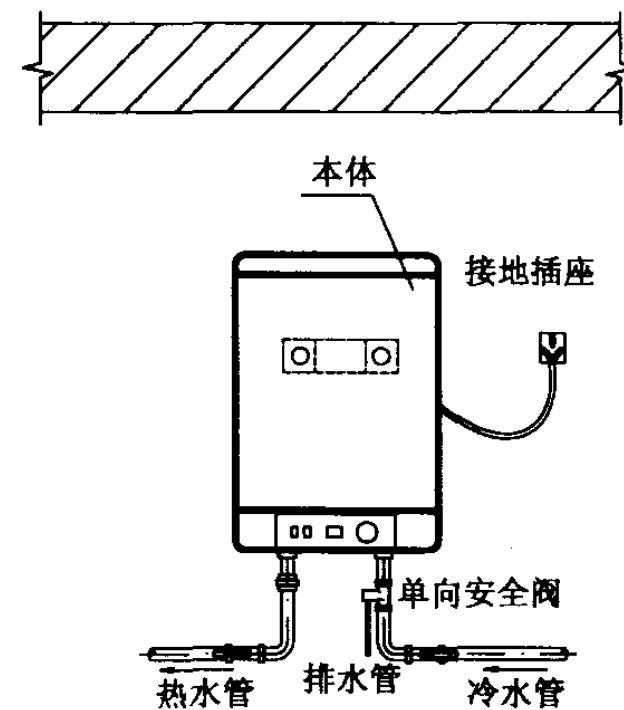
立面图(详)
