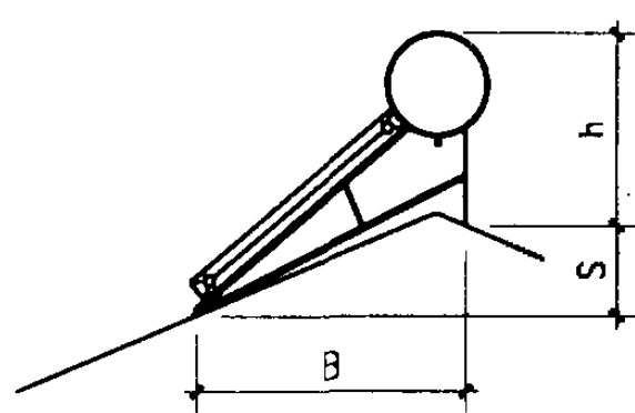
坡屋面屋脊安装
