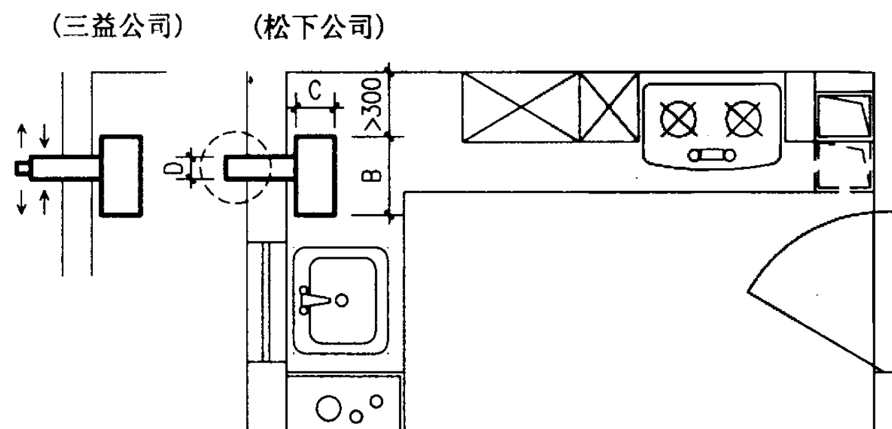
平面图
