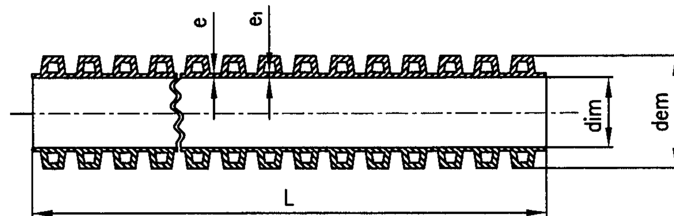
b) 不带扩口管材结构示意图
