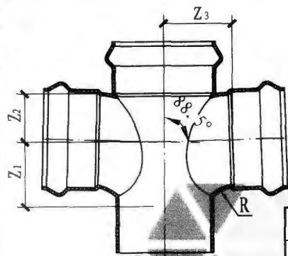
90° 带插口正四通
