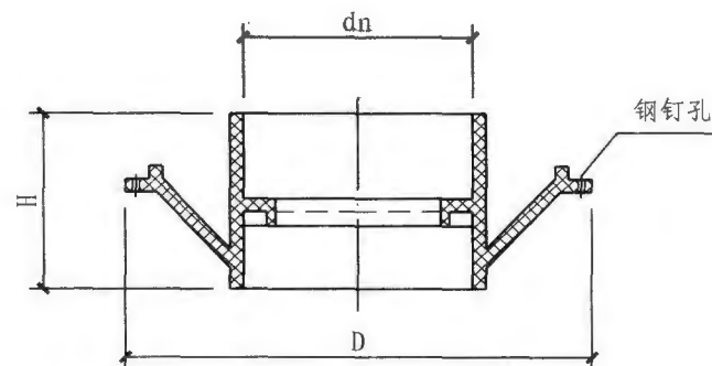
防渗套管构造图
