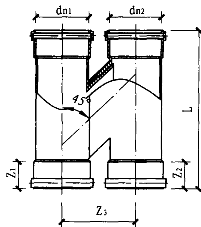
H管件
