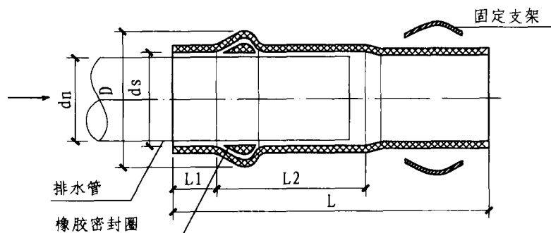
横管伸缩节剖面图
