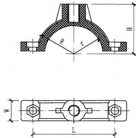
管夹
