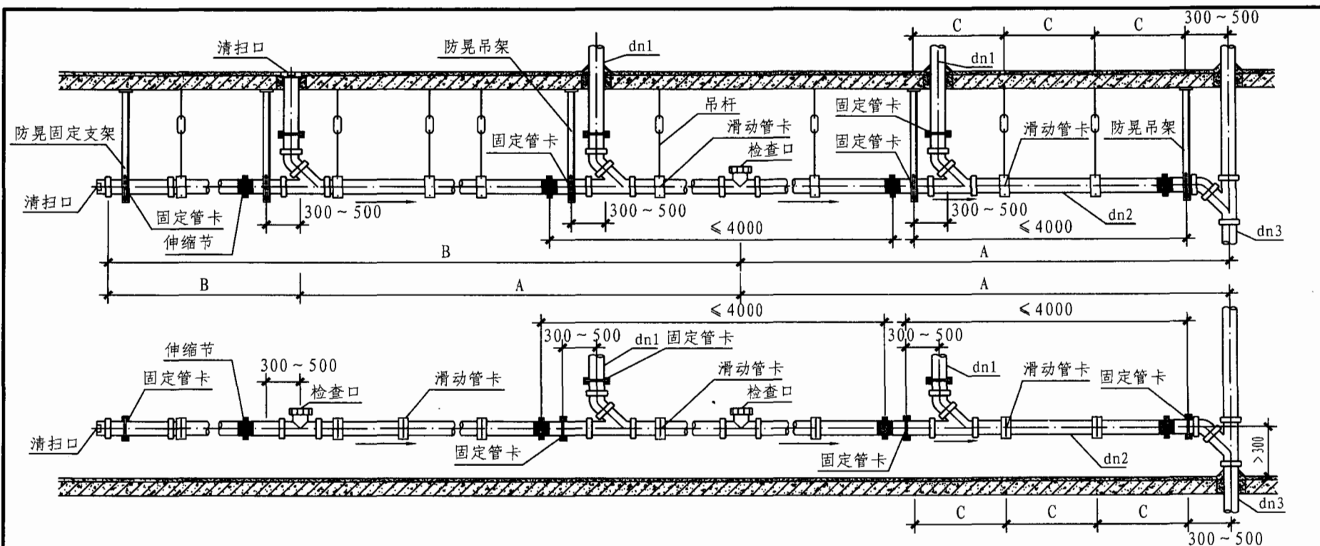
排水横管的直线管段检查口或清扫口 之间的最大距离和管道支、吊架最大间距及安装坡度
