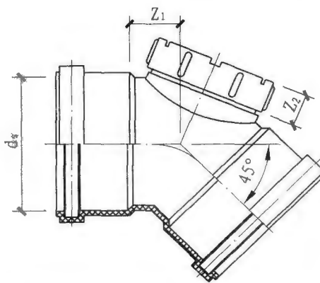
带检查口45° 弯头 (双承口)
