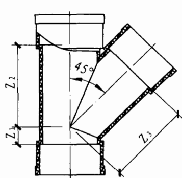
45° 斜三通
