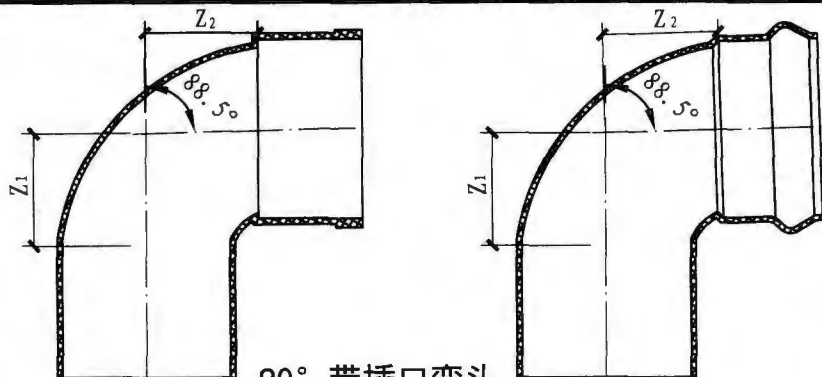
90° 带插口弯头
