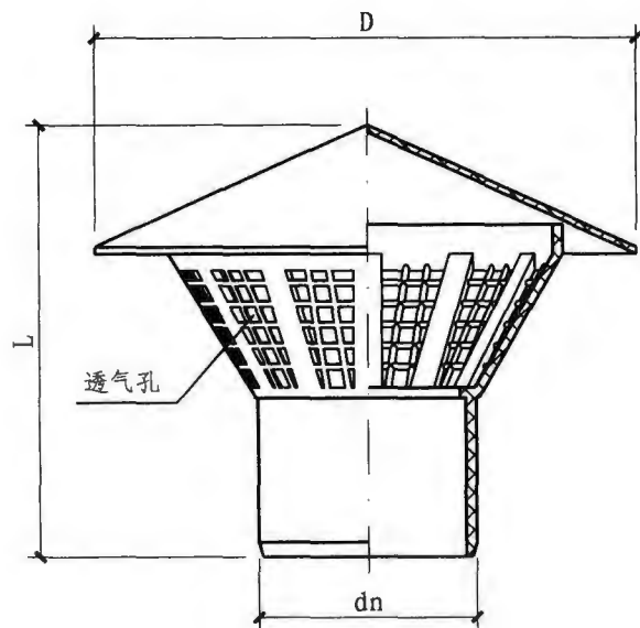
塑料通气帽
