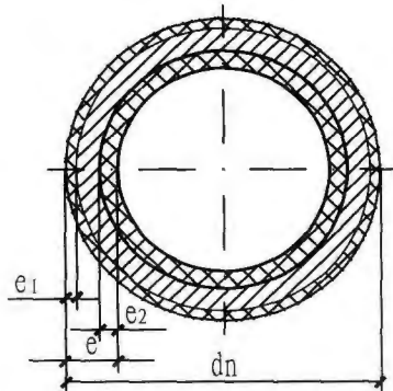
管材截面示意图
