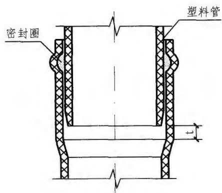
橡胶密封圈连接示意图
