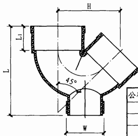
带检查口圆底存水弯
