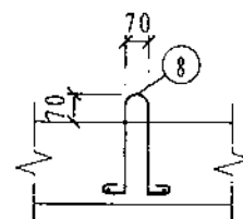
吊钩示意图
