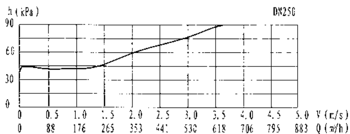
YQ系列减压型倒流防止器水头损失曲线
