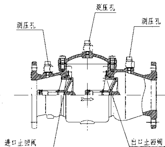
法兰连接双止回阀倒流防止器构造示意图
