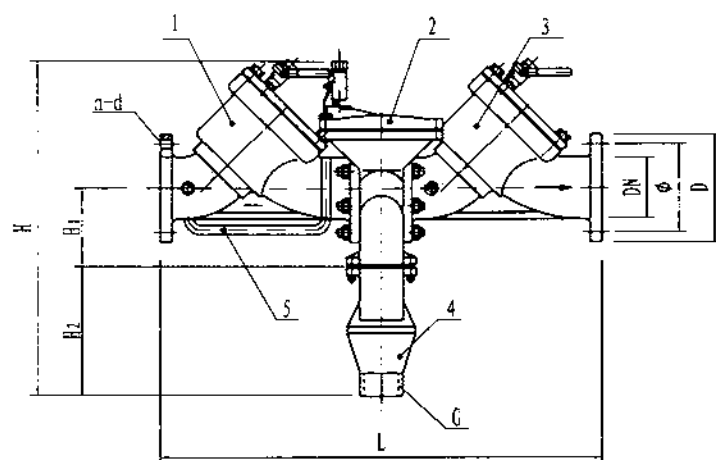
法兰连接减压型倒流防止器外形图
