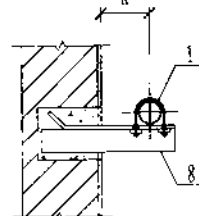
II-II剖面图 (托架)
