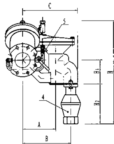
法兰连接减压型倒流防止器外形图
