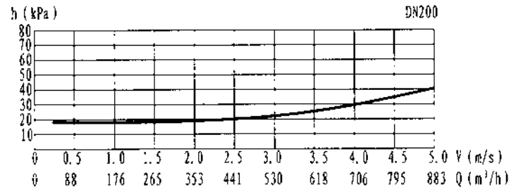
LHS743X型低阻力倒流防止器水头损失表 图集号
