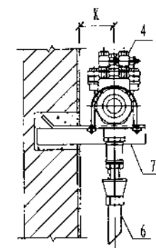
I-I剖面图
