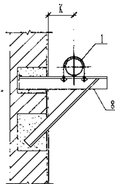
II-II剖面图
