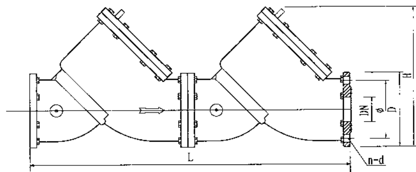
WT-709法兰连接倒流防止器外形图外形图
