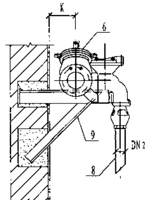
I-I剖面图
