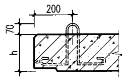
吊环安装示意
