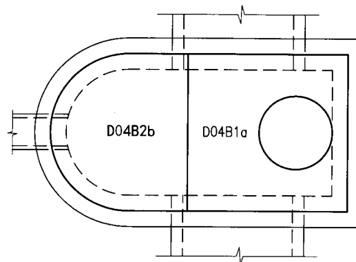
D04B2盖板布置图 (D=1000~1200)
