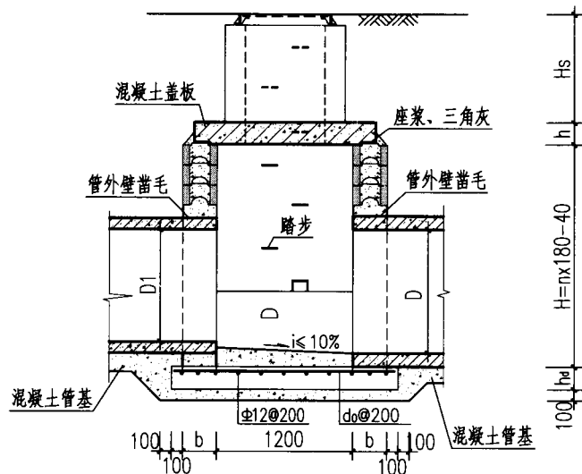
1-1剖面图
