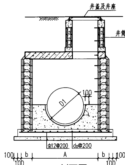
2-2剖面图
