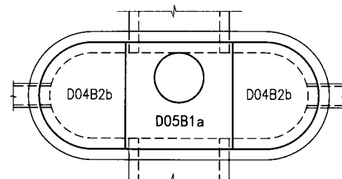
D05B3盖板布置图 (D=1300~1500)
