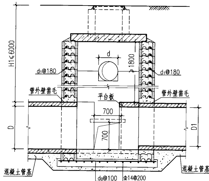
2-2剖面图
