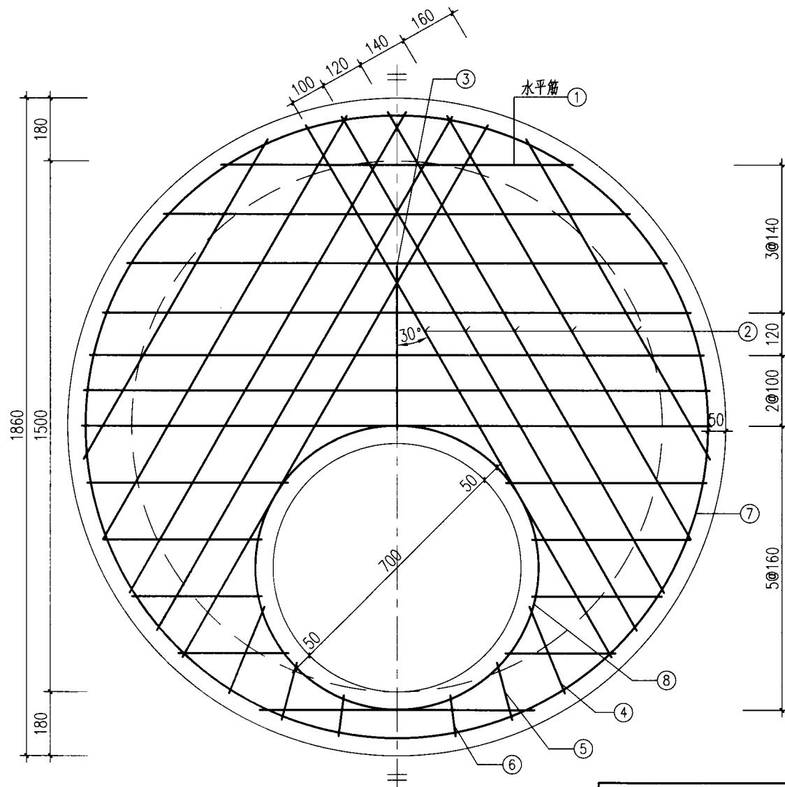
平面图
