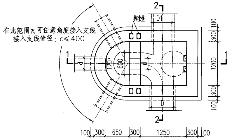
平面图
