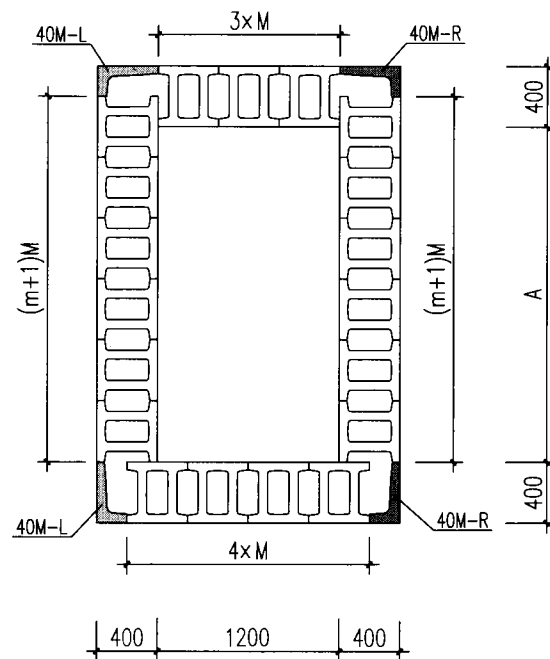
平面组砌图(偶数层)
