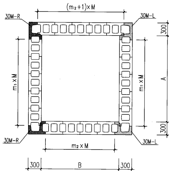
平面组砌图(奇数层)
