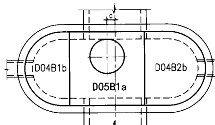
D05B2盖板布置图 (D=1000~1200)
