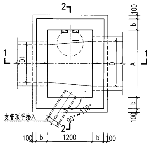
平面图
