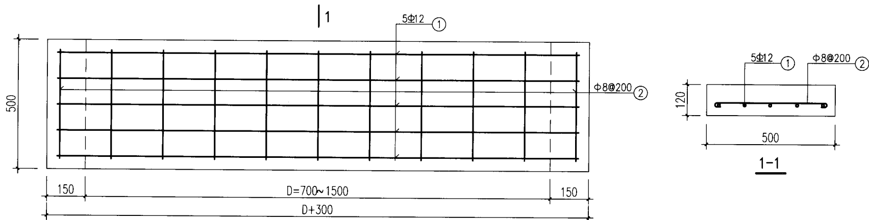
预制平台板平面图
