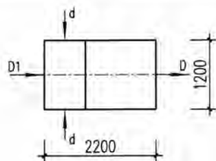
矩形竖槽式跌水井 (D01) (支、干管顺接)
