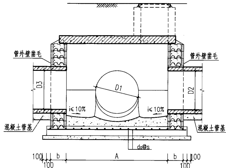
2-2 剖面图
