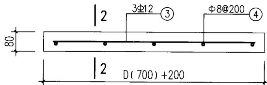
预制过梁
