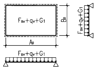
图1 盖板内力计算简图
