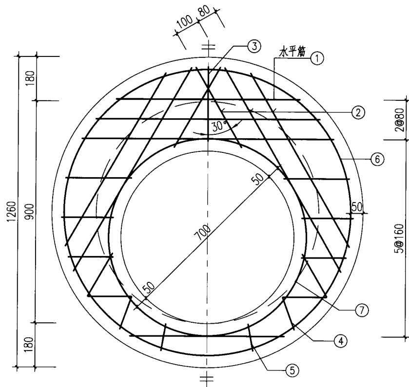
平面图
