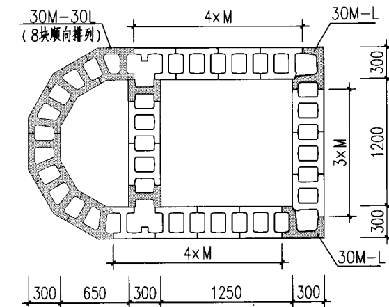
下部平面组砌图(偶数层)
