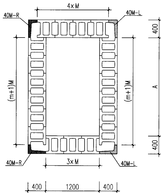
平面组砌图(奇数层)
