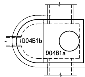
D04B1盖板布置图 (D=700~900)
