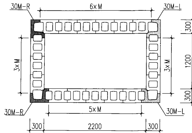
上部平面组砌图(偶数层)
