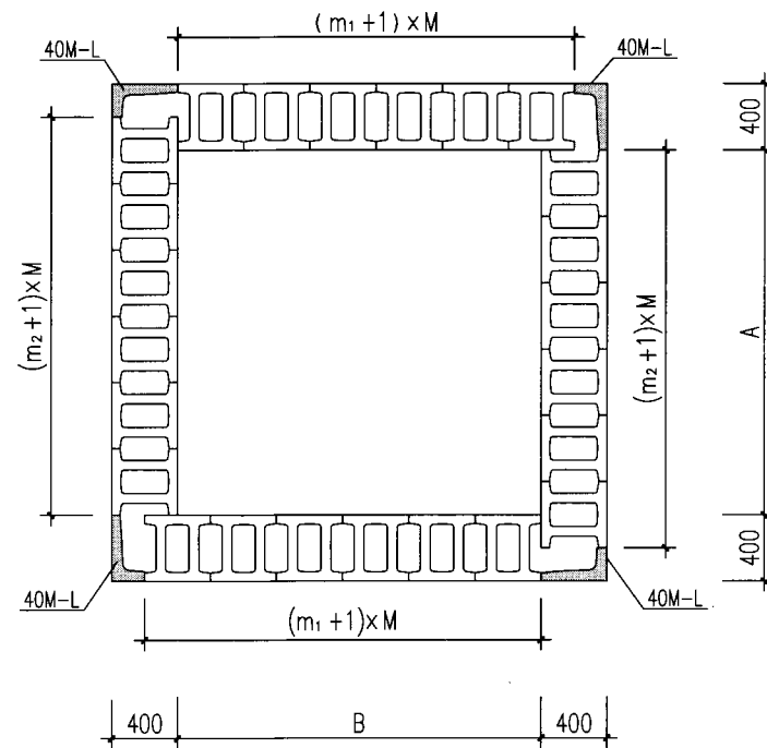
平面组砌图(偶数层)
