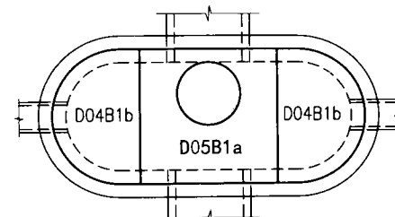
D05B1盖板布置图 (D=700~900)
