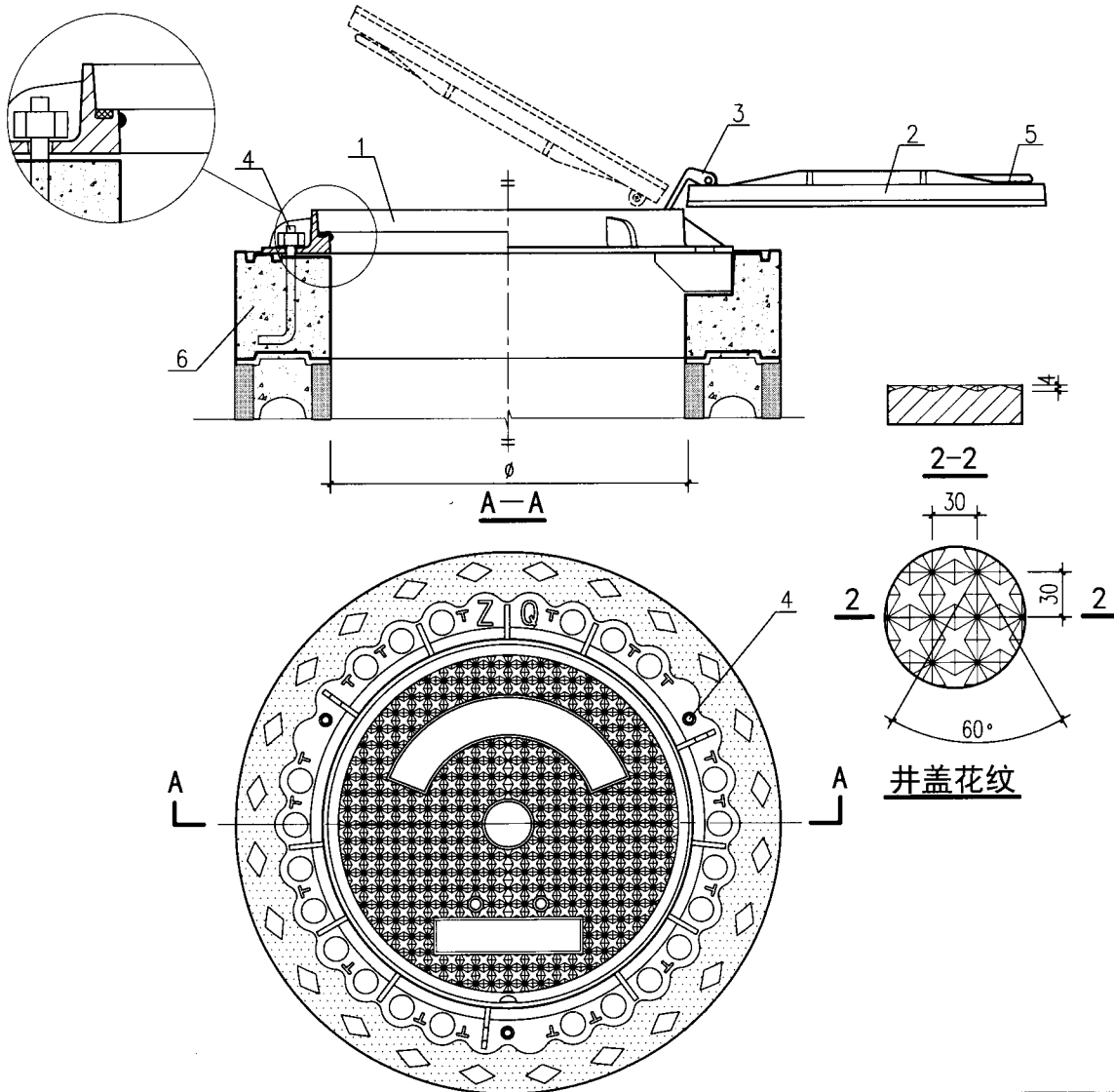
轻、重型铸铁井盖图
