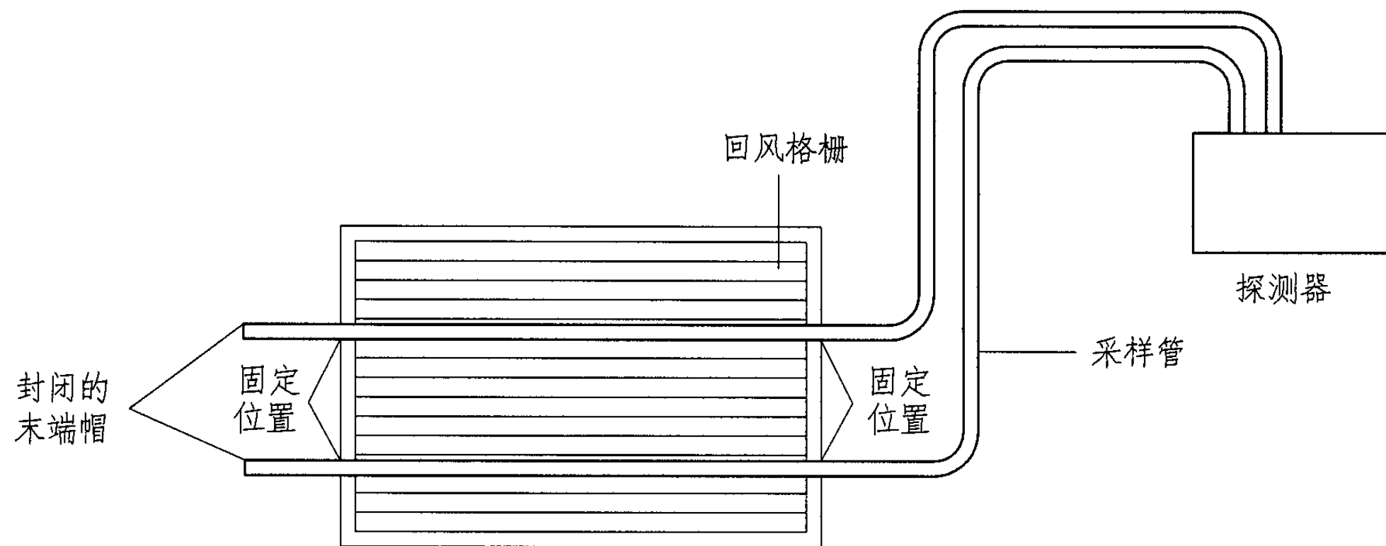
回风格栅采样示意图
