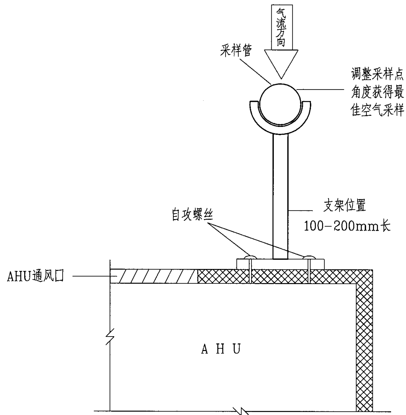
监控空气处理单元的采样管位置
