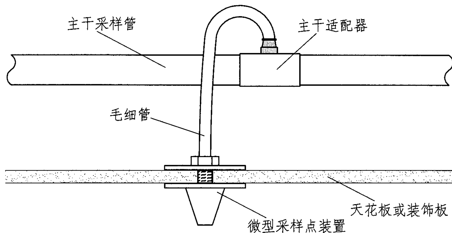
典型毛细管采样示意图
