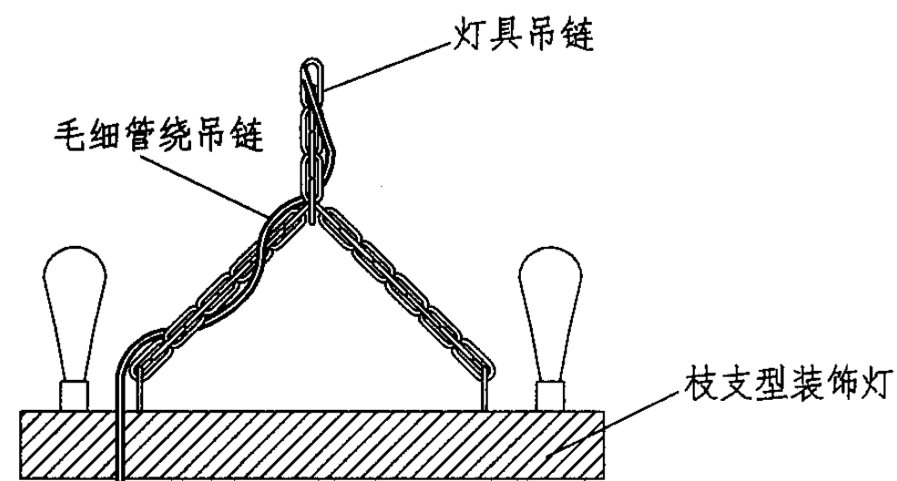
从装饰灯上采样示意图
