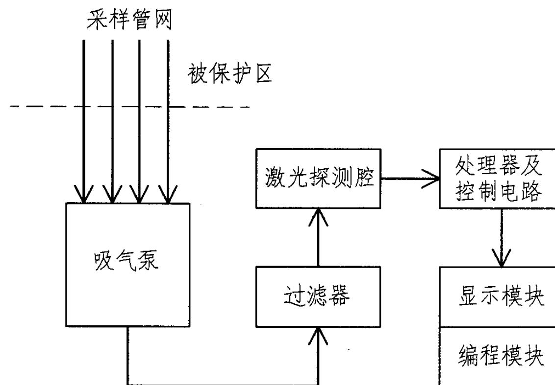
探测器工作原理方框图
