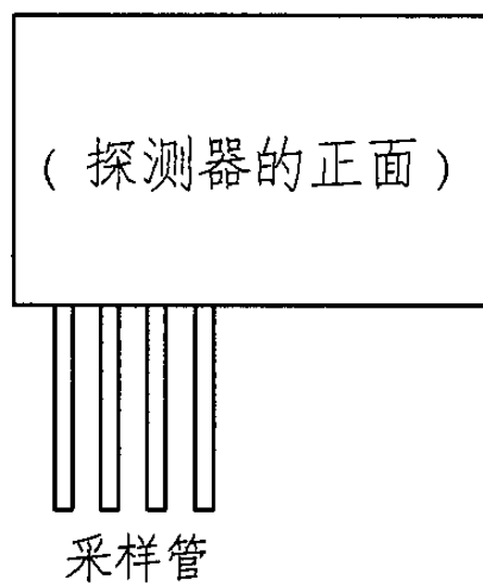
探测器的反向安装示意图
