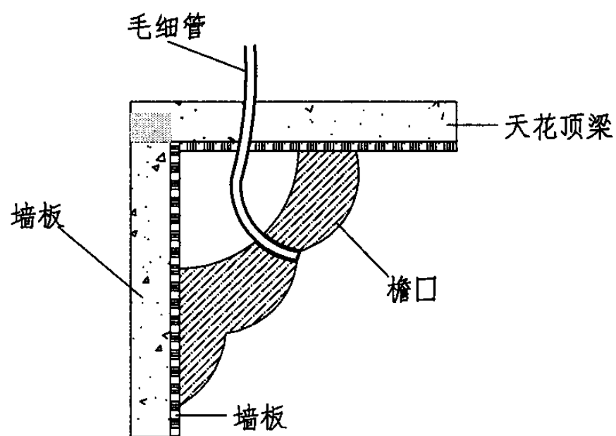
穿过檐口采样示意图
