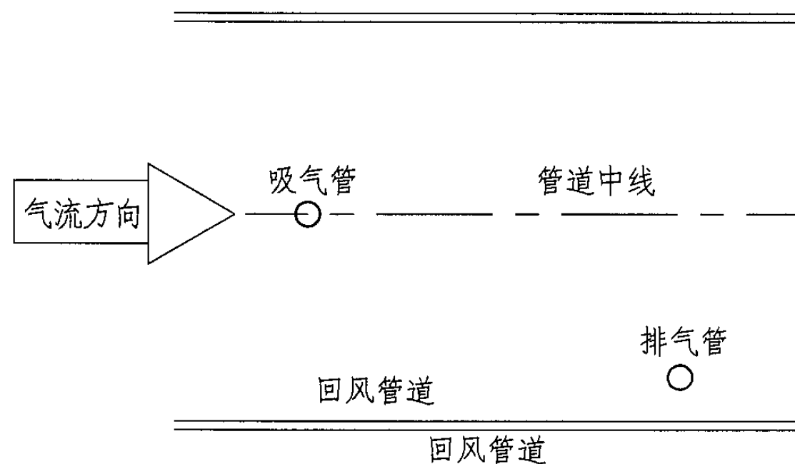
探测管及管道采样探测器的排列
