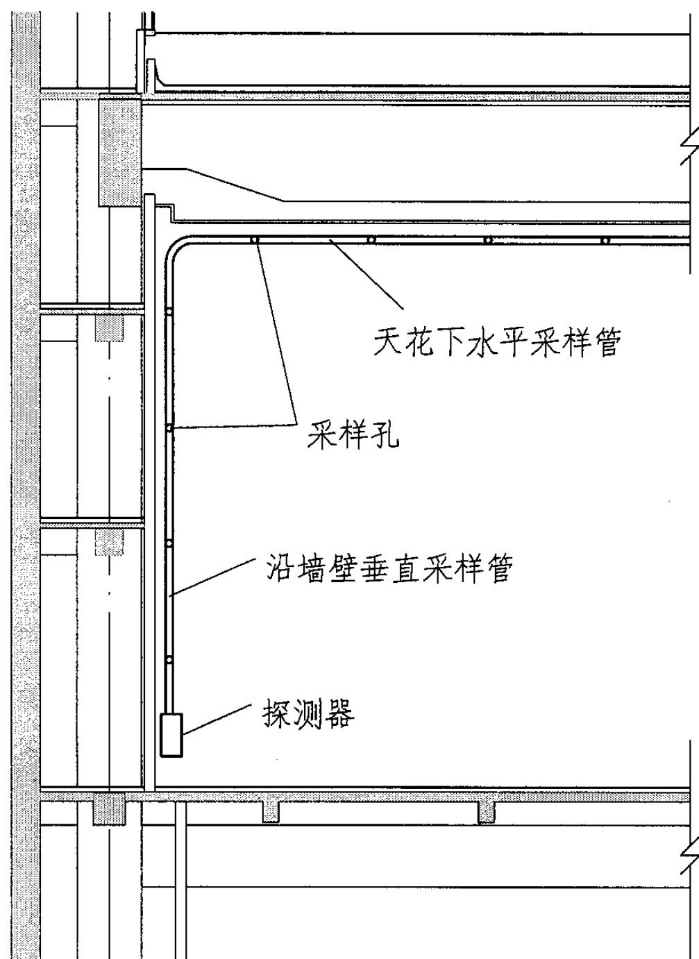
在高大宽敞的前厅内采样示意图
