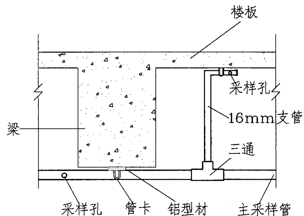
梁下手杖式采样示意图
