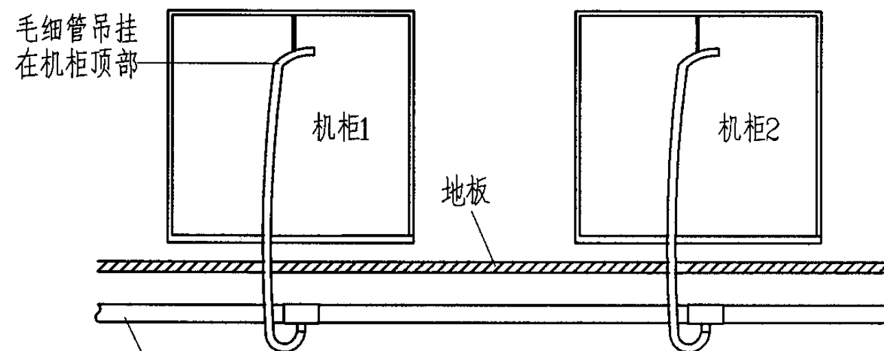
从地板下进行机柜内采样示意图
