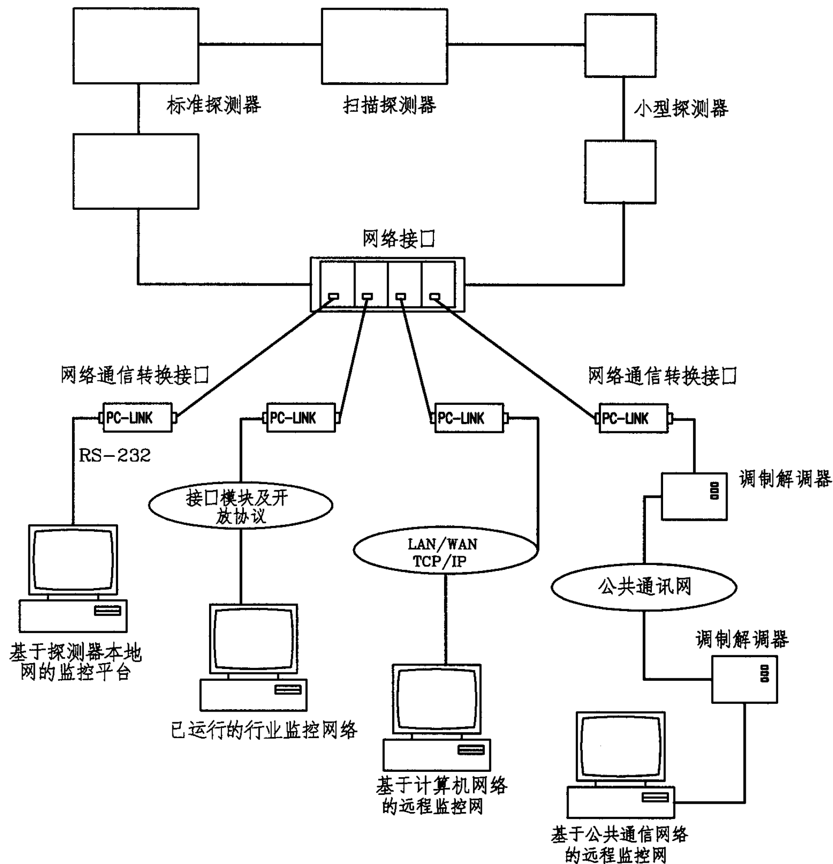
系统网络连接示意图
