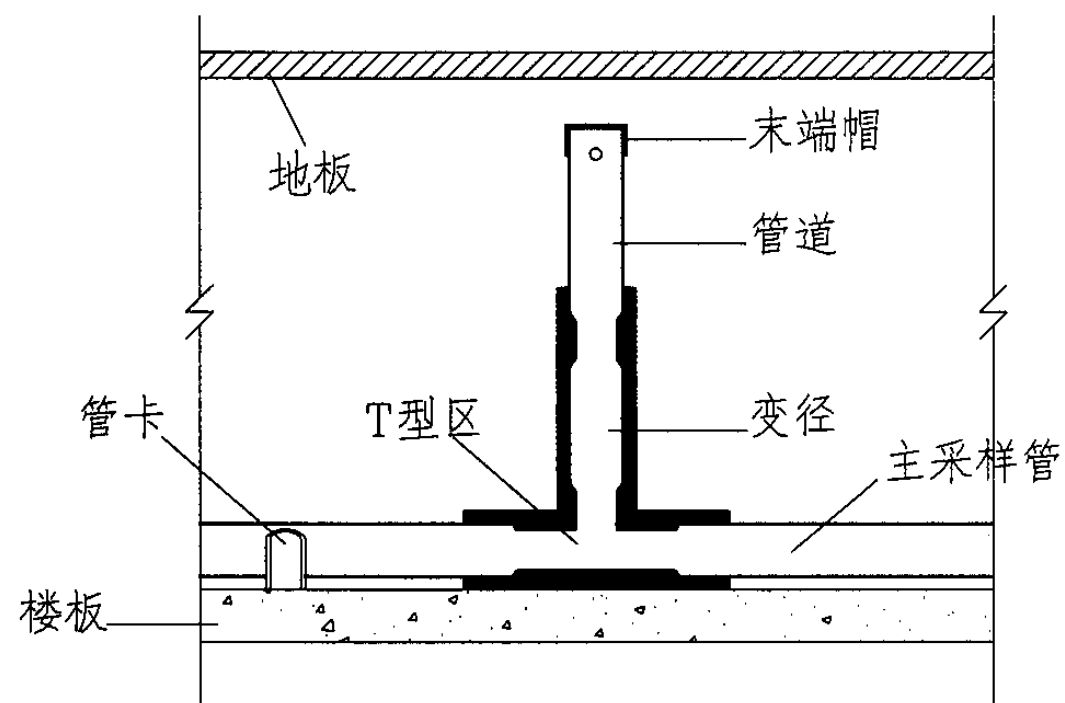
地板下的立式管道采样示意图
