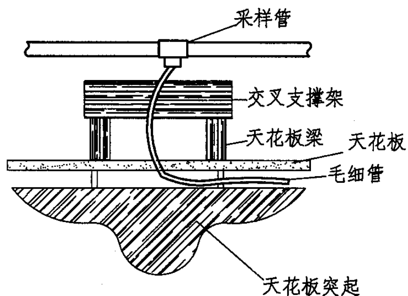
天花板下突起处采样示意图
