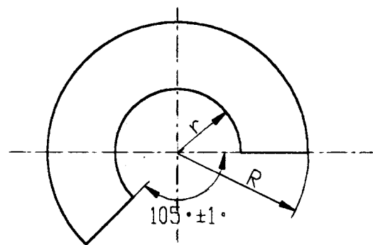
锥形罩展开图
