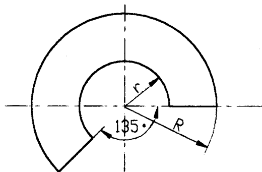
锥形罩展开图
