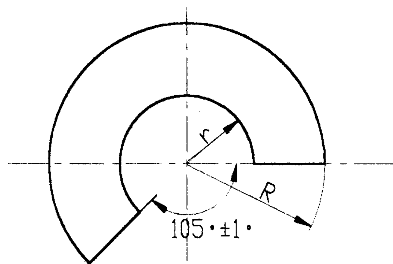
锥形罩展开图
