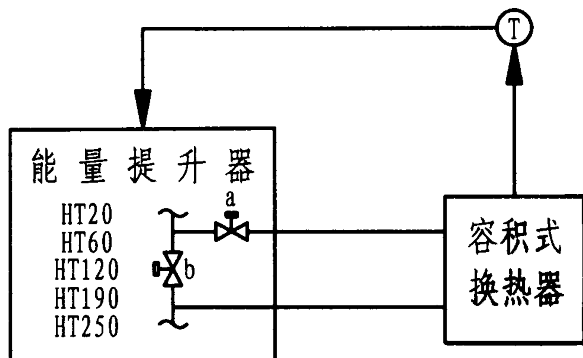
单台换热器热水控制
