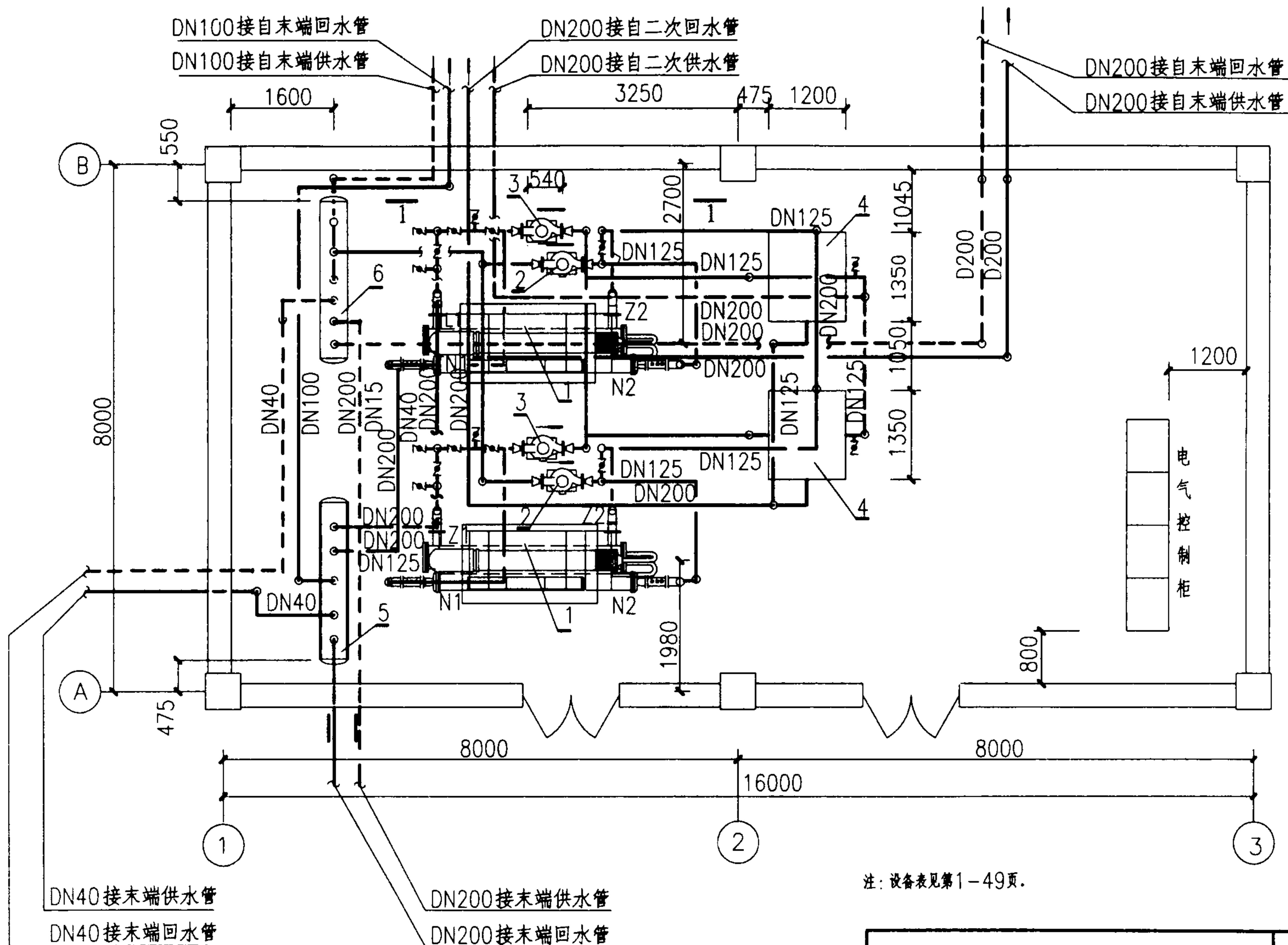
HT760(二台) 冷热源设备及管道平面图
