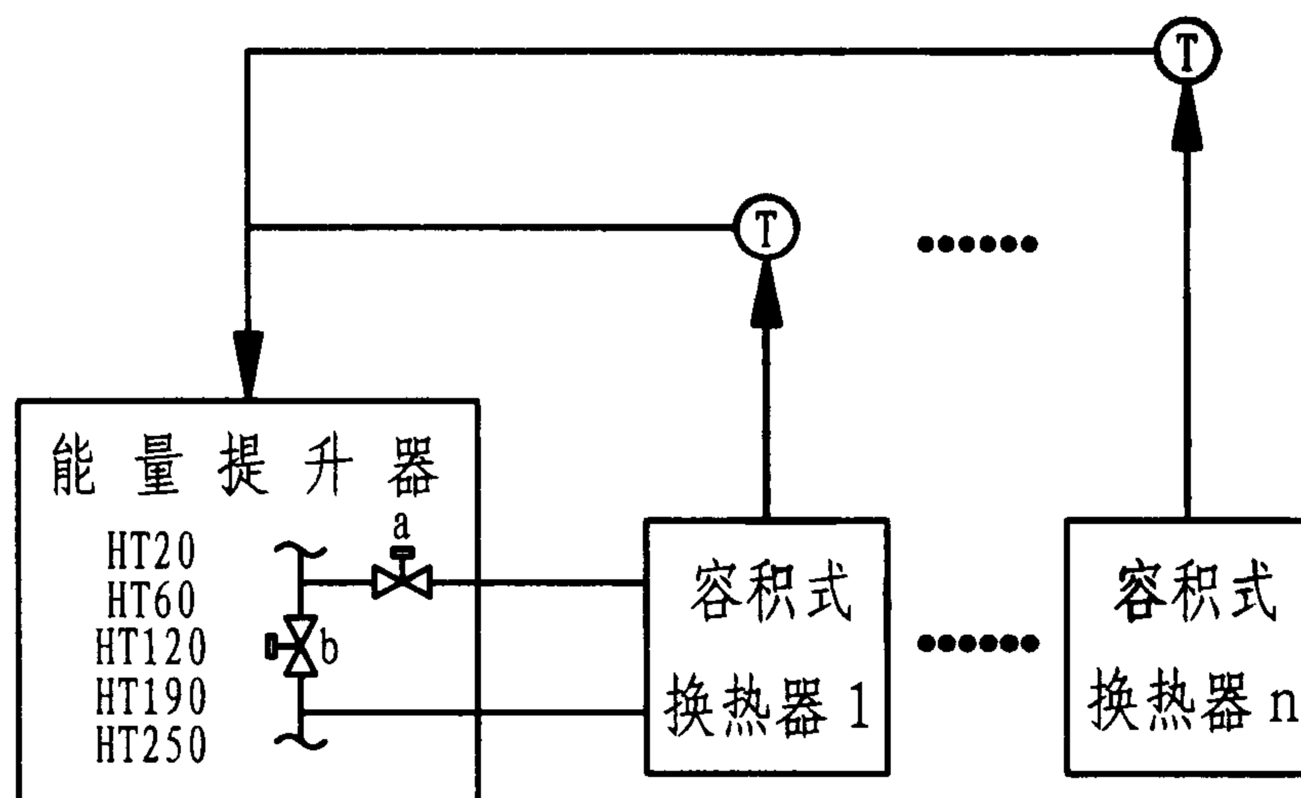
多台换热器热水控制
