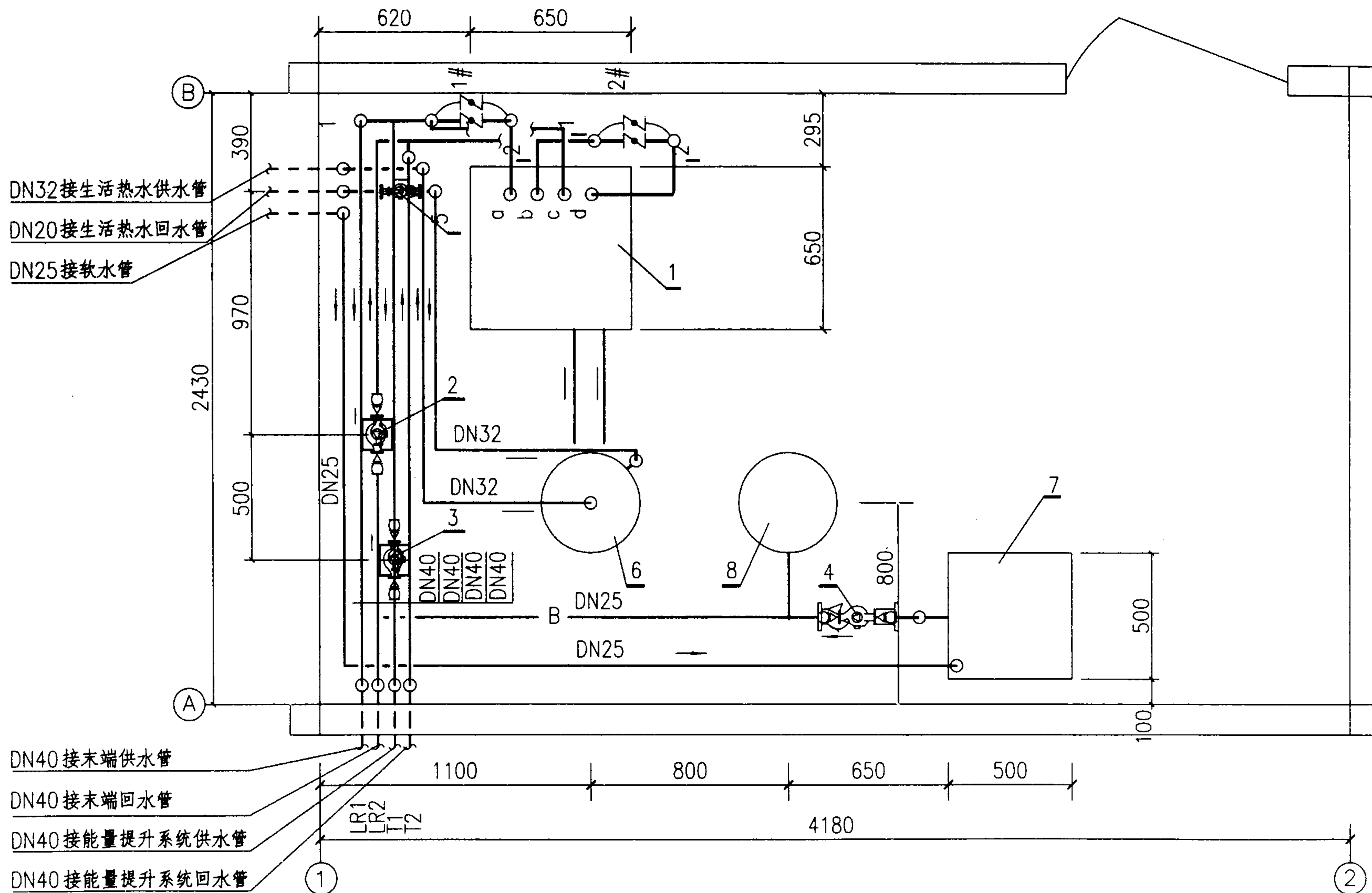
HT60(一台)冷热源设备及管道平面图
