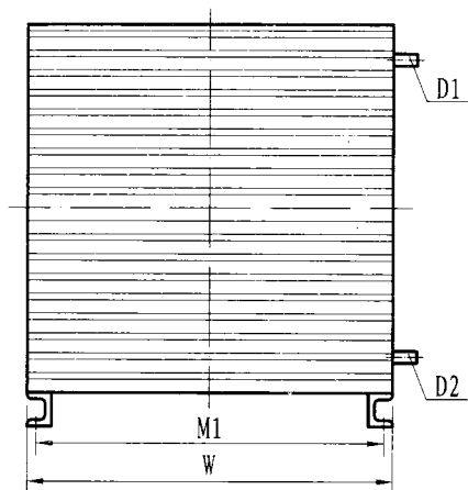
立面图
