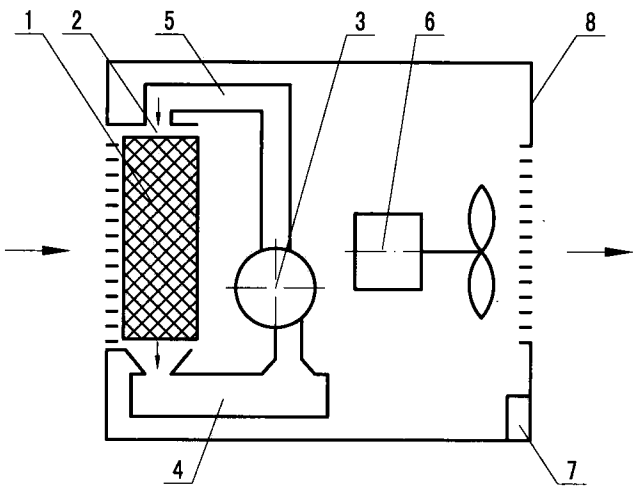
图1 工作原理图
