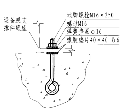
④ 橡胶垫片安装
