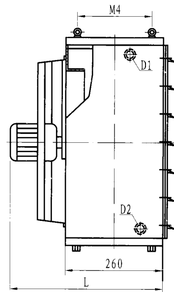
侧面图
