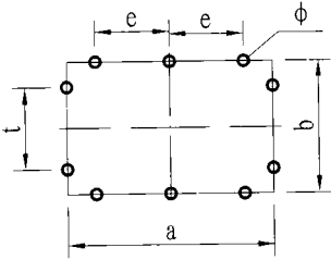
基础螺孔位置图
