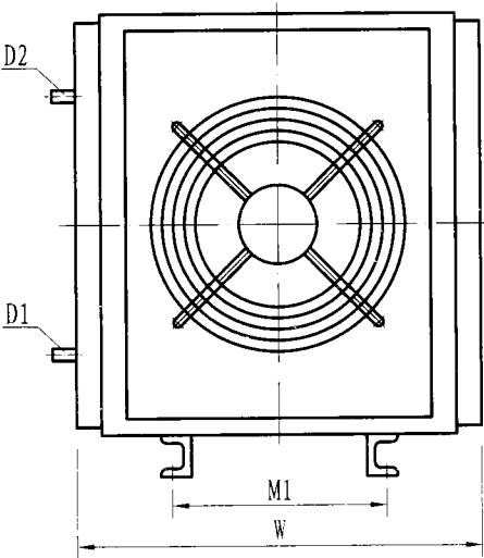
立面图
