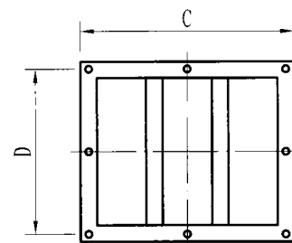
底座平面图
